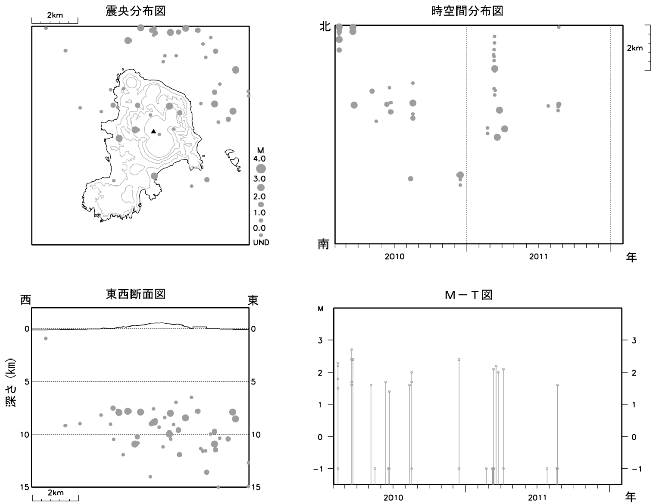
図 4 ※ 神津島 広域地震観測網による山体・周辺の地震活動（2010 年 2 月 1 日～2012 年 1 月 31 日）
