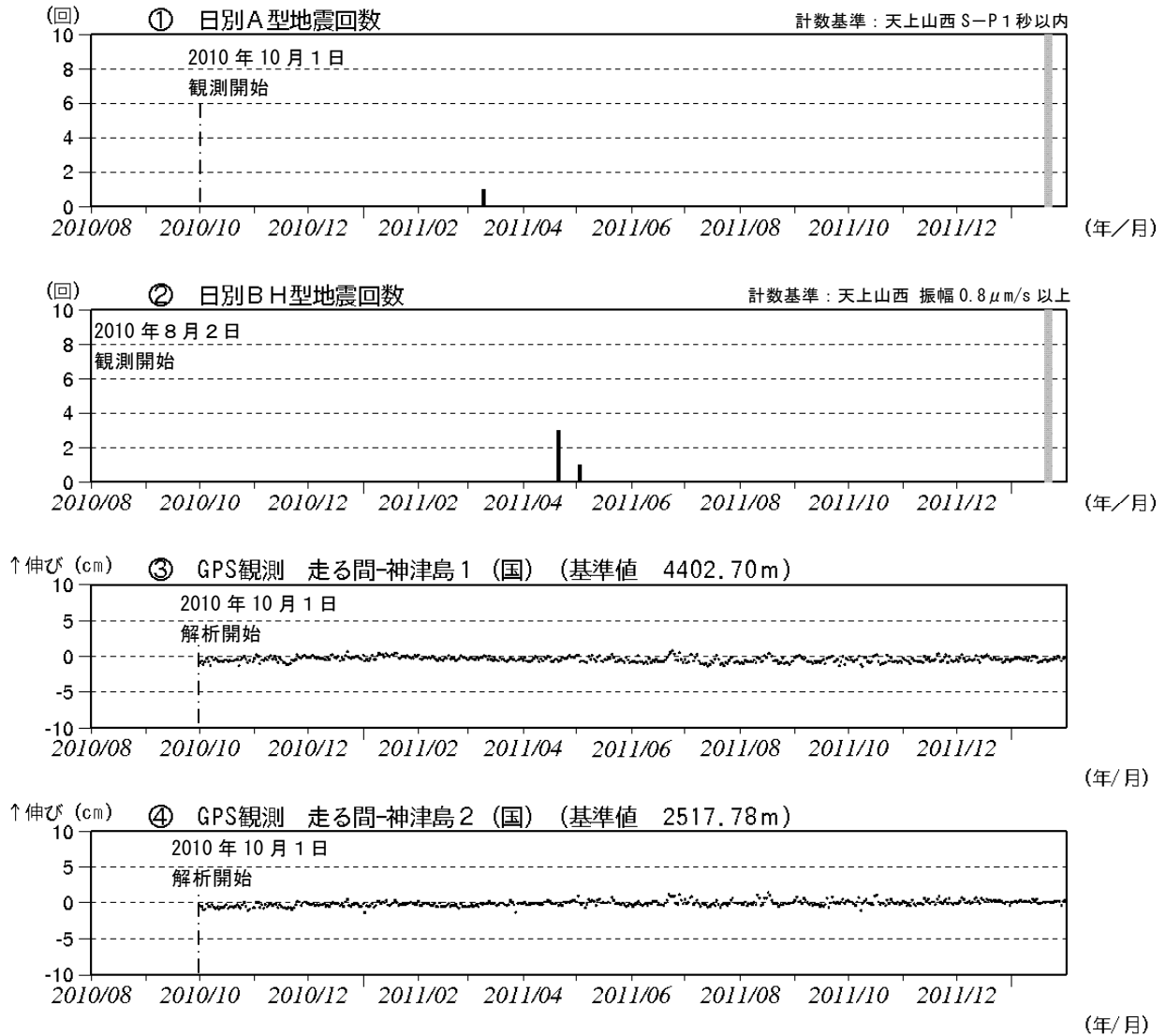
図 3 神津島 火山活動経過図(2010 年 8 月～2011 年 12 月)
