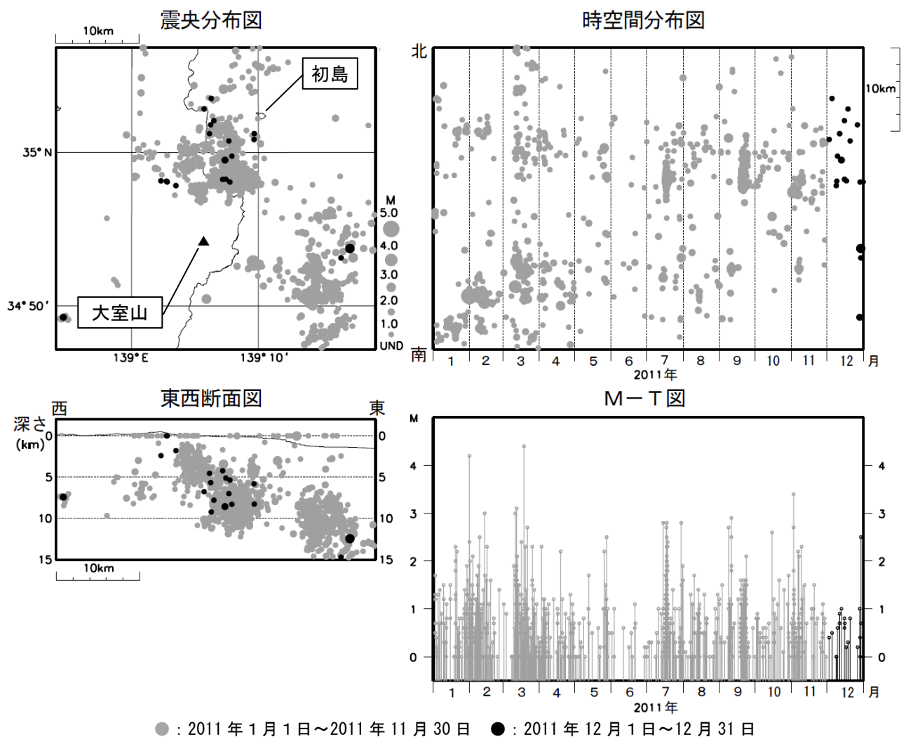
図 2※ 伊豆東部火山群 広域地震観測網による震源分布図（2011 年 1 月 1 日～2011 年 12 月 31 日） M（マグニチュード）は地震の規模を表します。 2011 年 3～5 月は一部未処理の期間があります。 図中の震源要素は一部暫定値が含まれており、後日変更することがあります。
