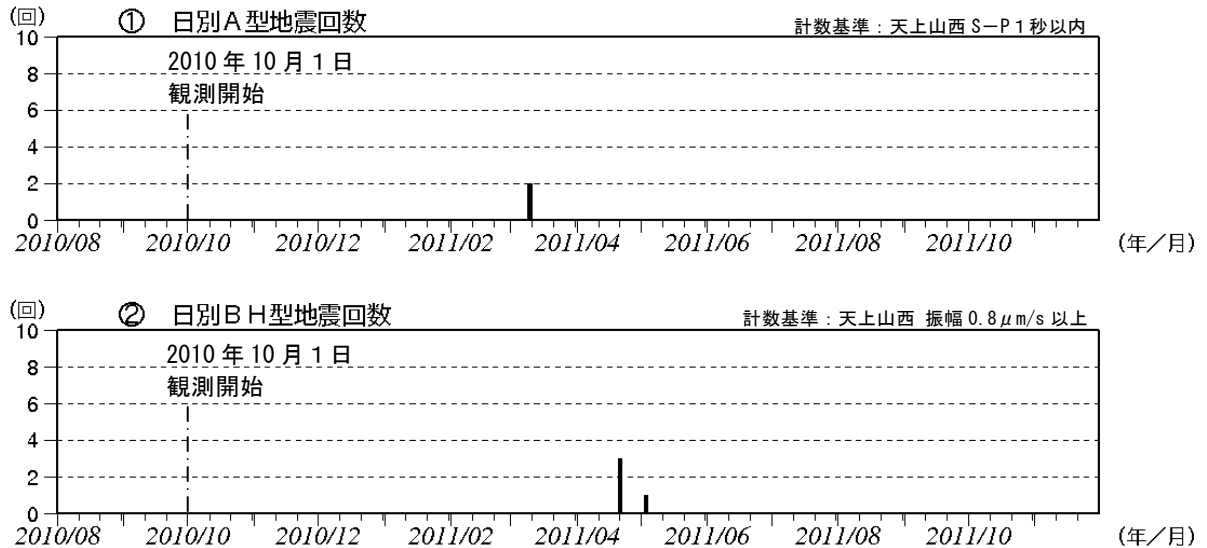
図3 神津島 日別地震回数(2010年10月～2011年11月) 3月～5月分は一部未処理の期間があります。
