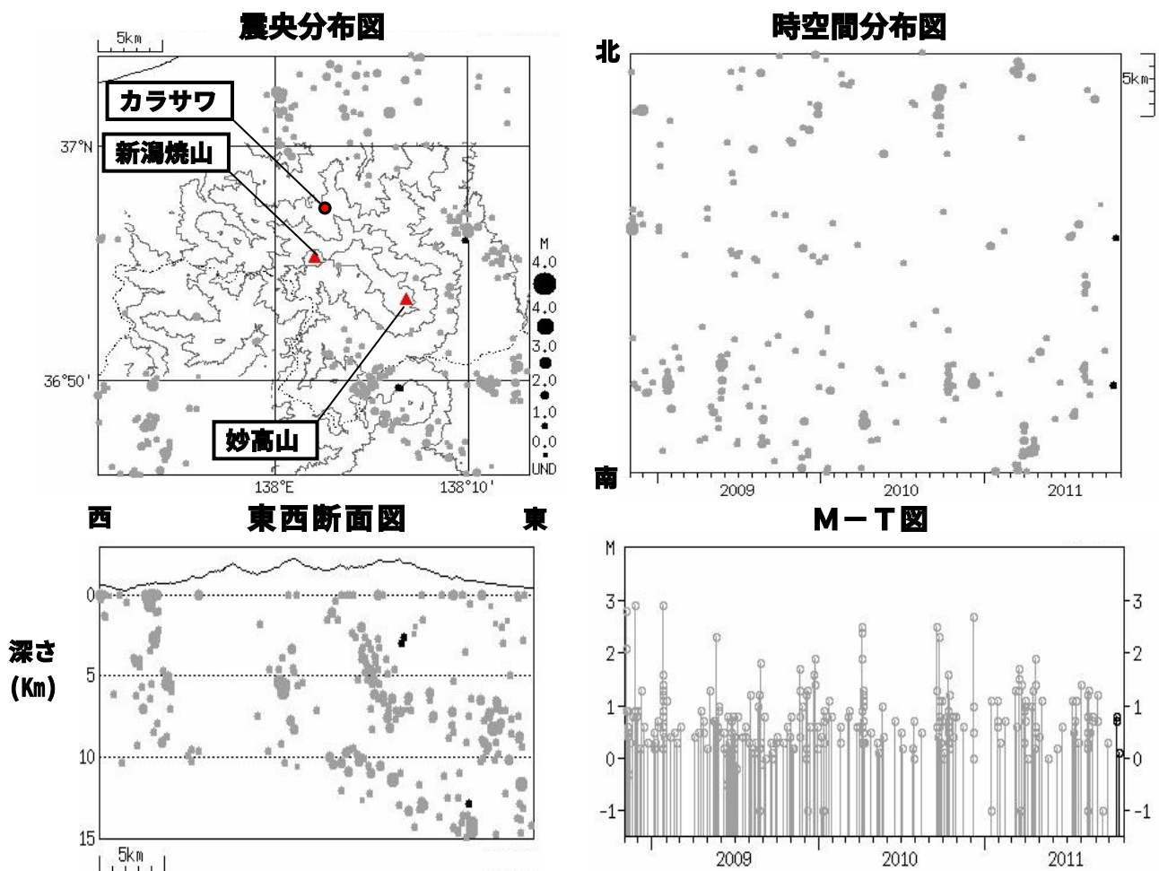
図4※ 新潟焼山 広域地震観測網による山体・周辺の地震活動(2008年11月1日～2011年10月31日)
