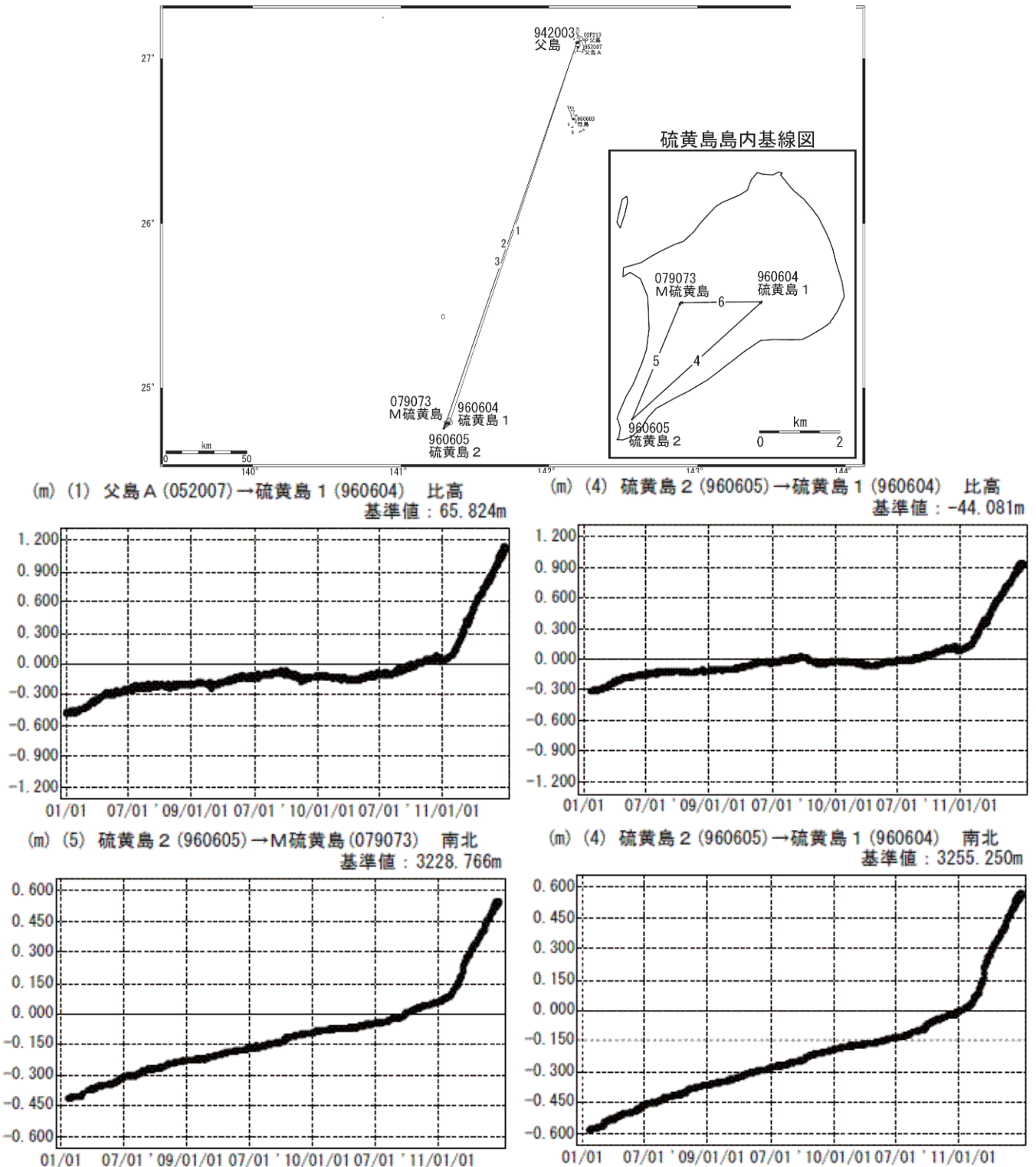
図 3※ 硫黄島 国土地理院による GPS 観測結果 1) （2008 年 1 月 1 日～2011 年 6 月 28 日）
