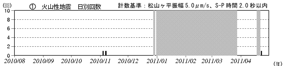
図 3 青ヶ島 火山性地震日別回数（2010 年 8 月 1 日～2011 年 4 月 30 日）
