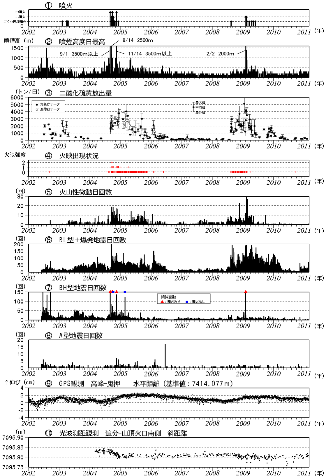
図3※ 浅間山 最近の火山活動の推移 (2002年1月1日~2011年2月28日)
