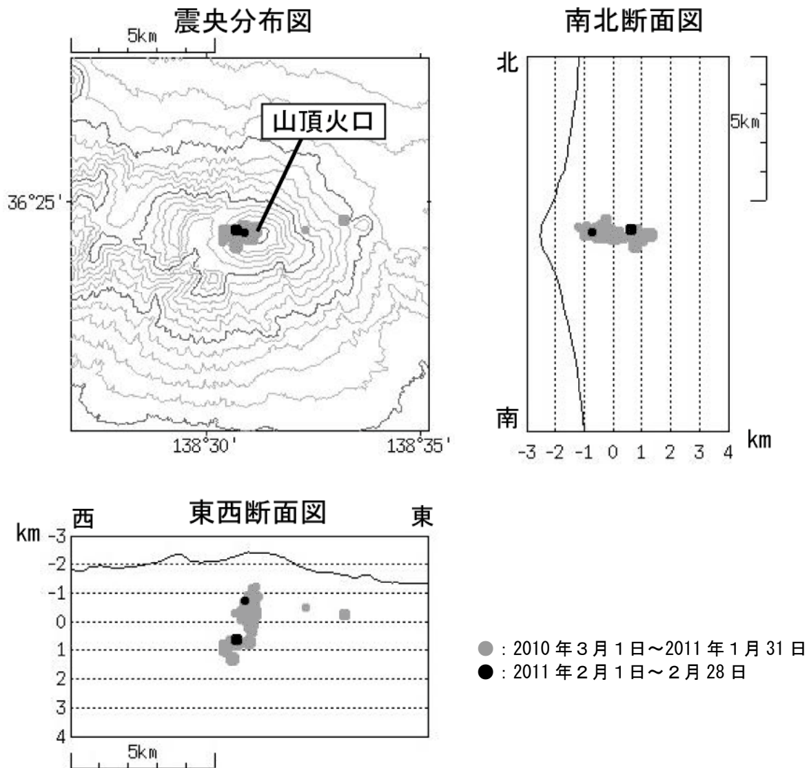
図 4 ※ 浅間山 震源分布図（2010 年 3 月 1 日～2011 年 2 月 28 日）
