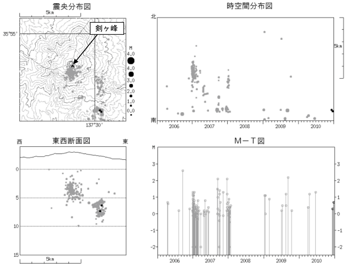
図 4※ 御嶽山 震源分布図（2006 年 1 月 1 日～2010 年 12 月 31 日）
