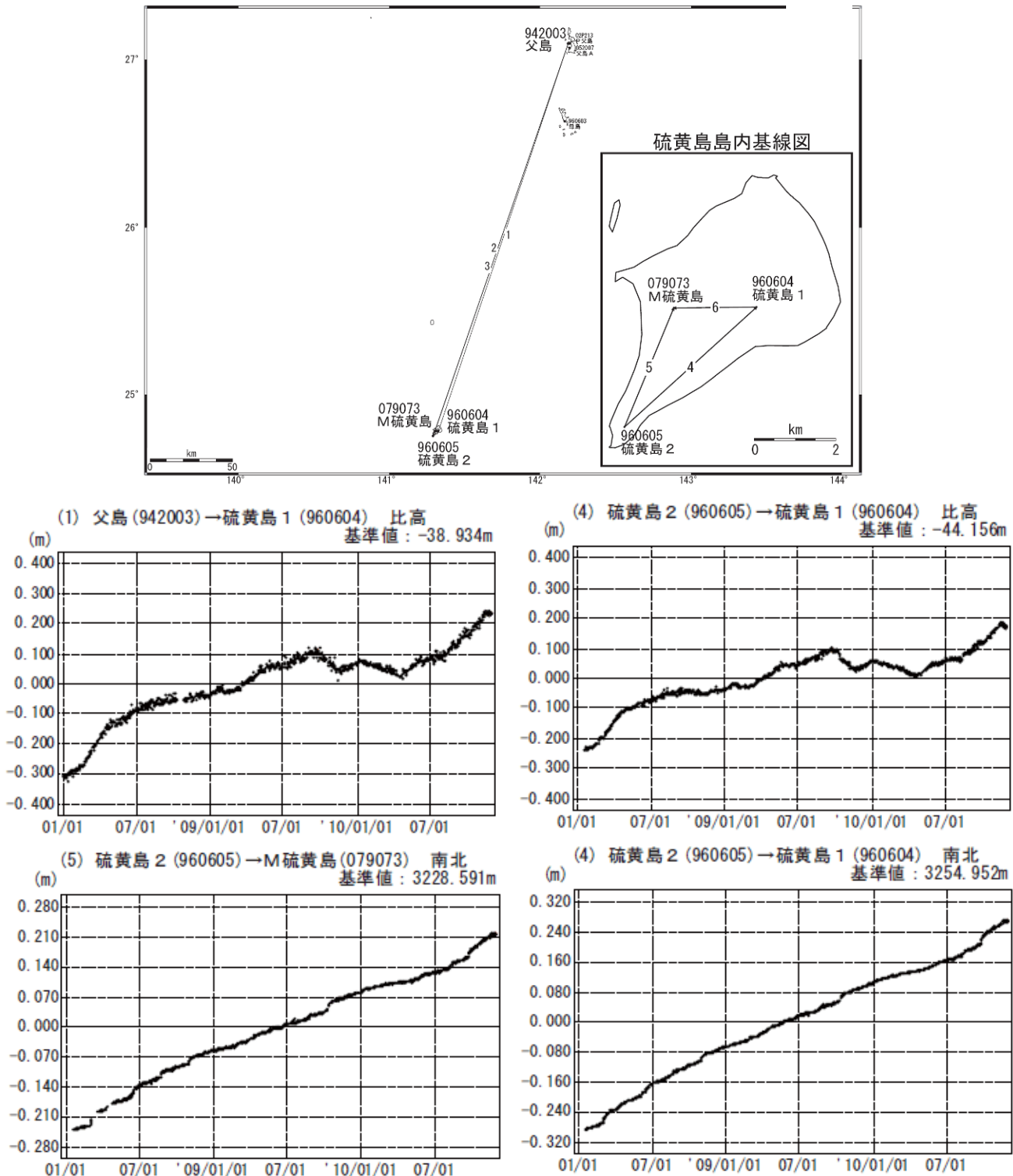
図 1 ※ 硫黄島 国土地理院による GPS 観測結果 1) (2008 年 1 月 1 日～2010 年 11 月 29 日)
