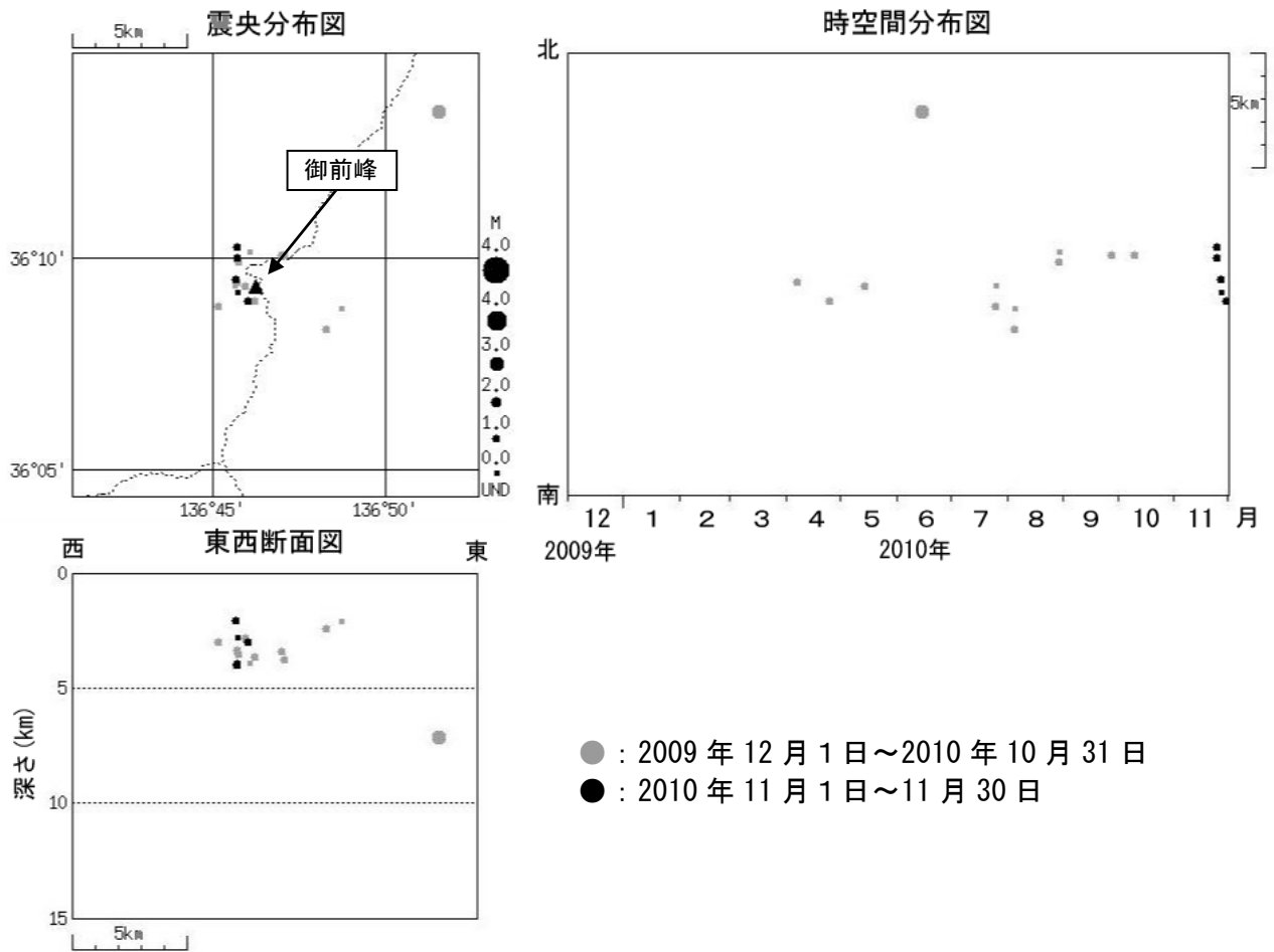
図 3※ 白山 震源分布図（2009 年 12 月 1 日～2010 年 11 月 30 日）
