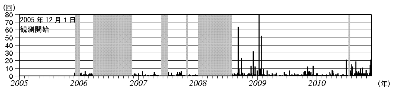
図 2 白山 日別地震回数（2005 年 12 月 1 日～2010 年 11 月 30 日）
