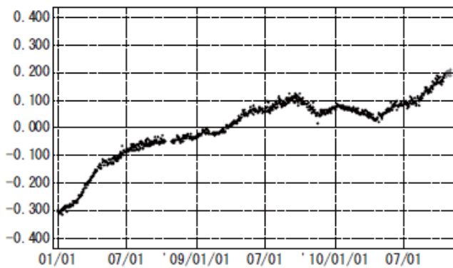
(m) (5) 硫黄島 2 (960605) → M硫黄島 (079073) 南北 基準値：3228.585m
