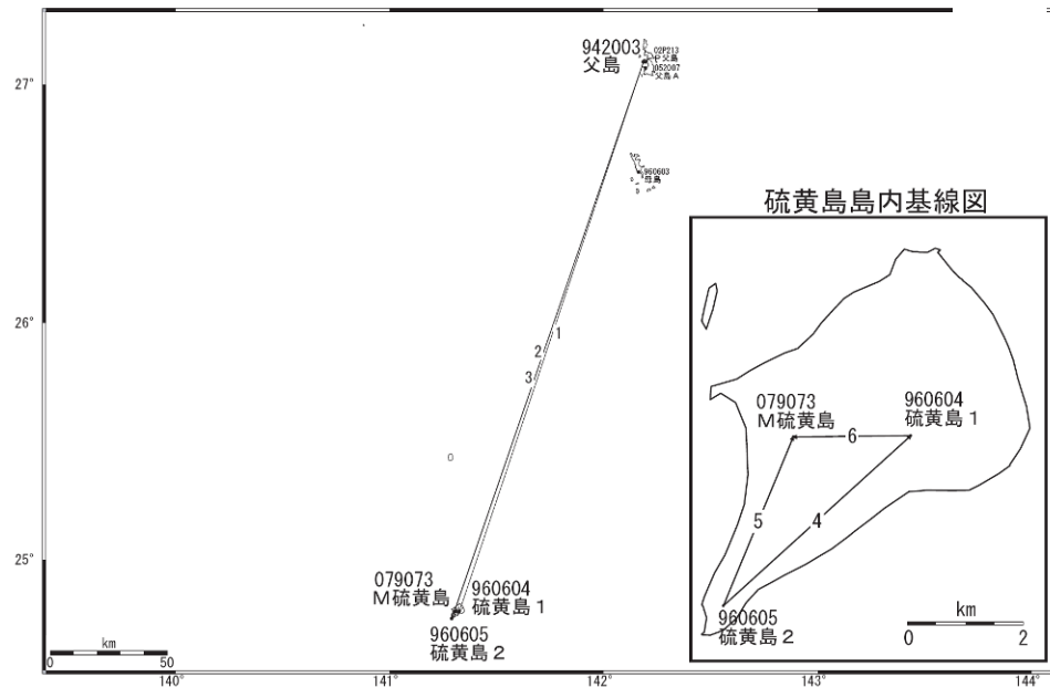
(m) (1) 父島 (942003) → 硫黄島 1 (960604) 比高 基準値：-38.940m
