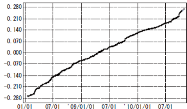
図 1※ 硫黄島 国土地理院による GPS 観測結果 1) (2008 年 1 月 1 日～2010 年 10 月 31 日)
