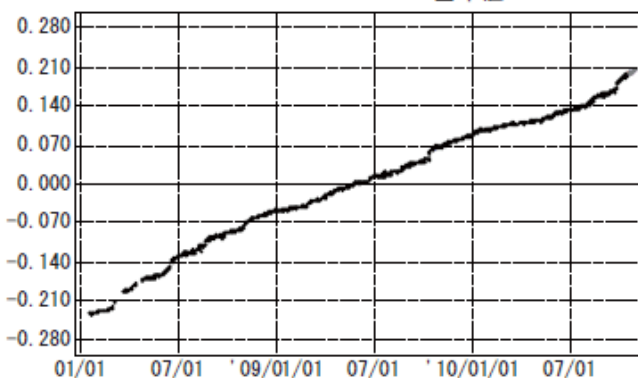
図 1※ 硫黄島 国土地理院による GPS 観測結果 1) (2008 年 1 月 1 日～2010 年 10 月 31 日)
