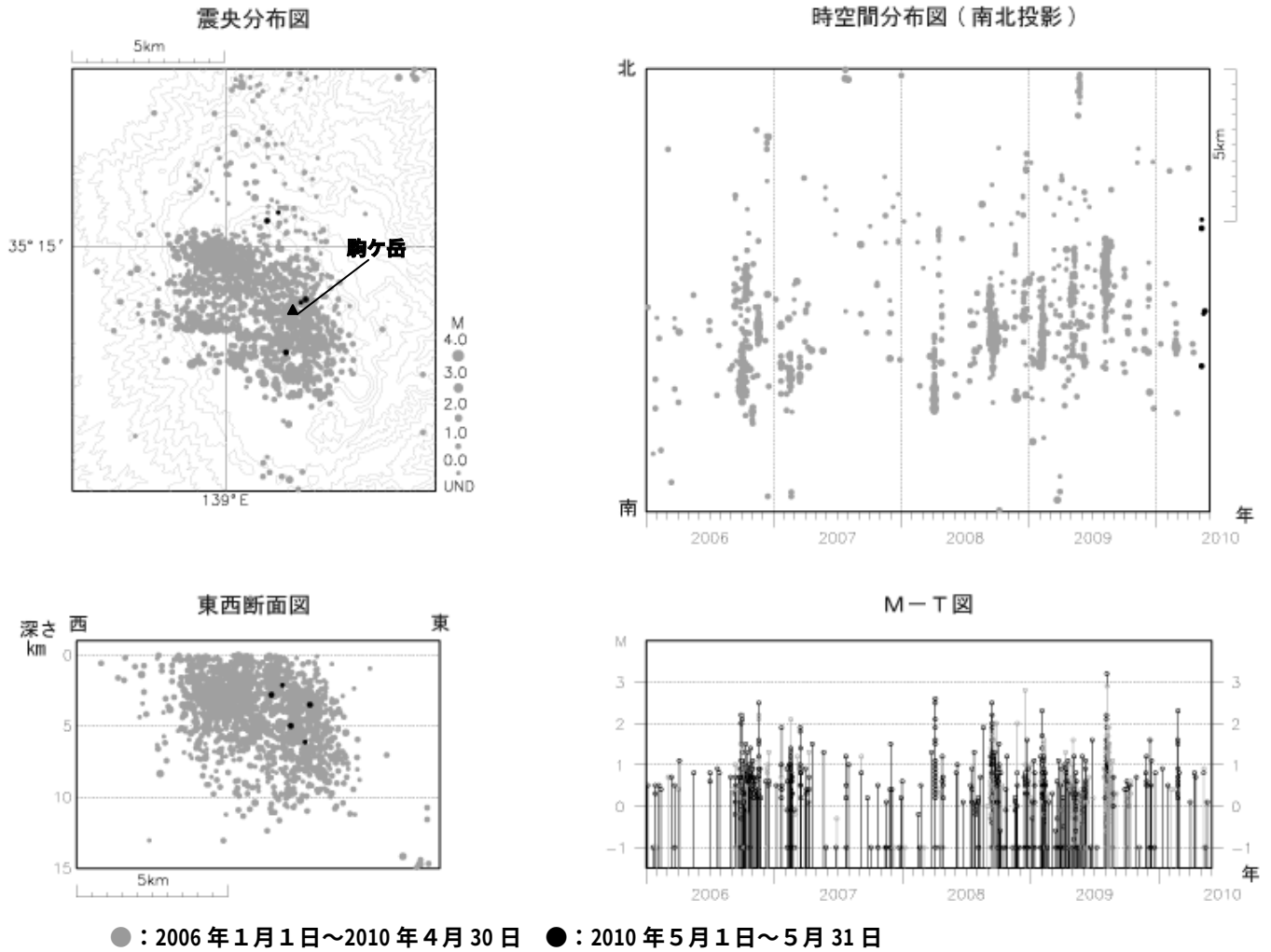
図 4 ※ 箱根山 震源分布図 (2006 年 1 月 1 日 ~ 2010 年 5 月 31 日) M (マグニチュード) は地震の規模を表します。 図中の震源要素は一部暫定値が含まれており、後日変更することがあります。
