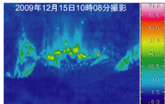
図1 伊豆大島 三原山山頂火口内及び山頂部の状況 円内は剣ガ峰付近のごく弱い噴気
