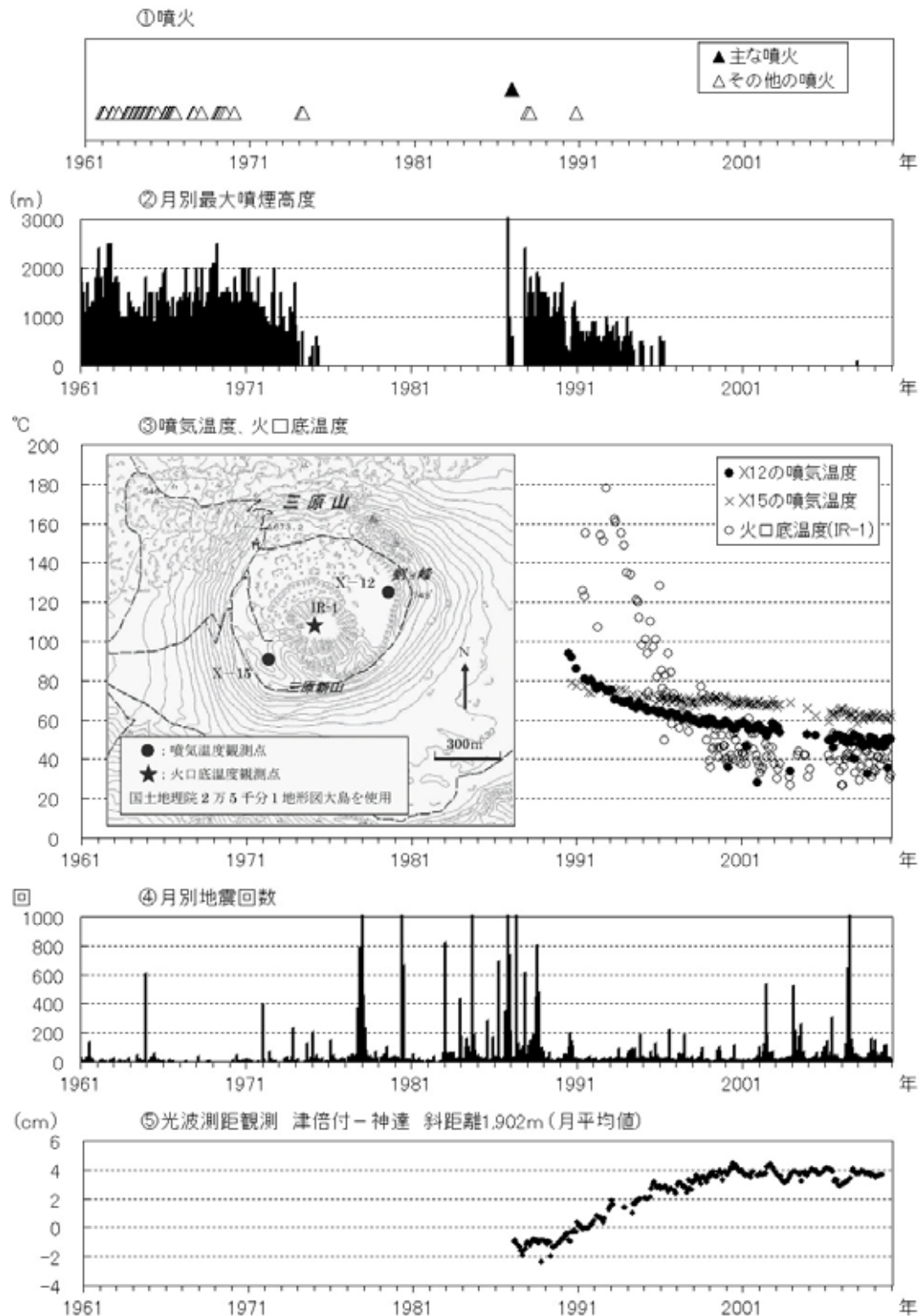
図4 伊豆大島 長期間の火山活動経過図（1961年1月～2010年1月）
