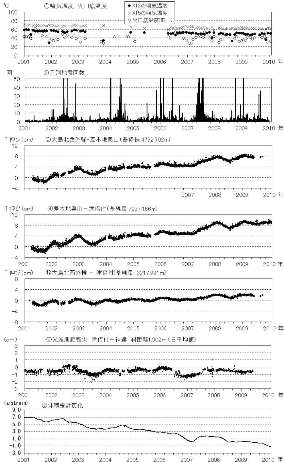
図5 伊豆大島 最近の火山活動経過図（2001年1月～2010年1月）
