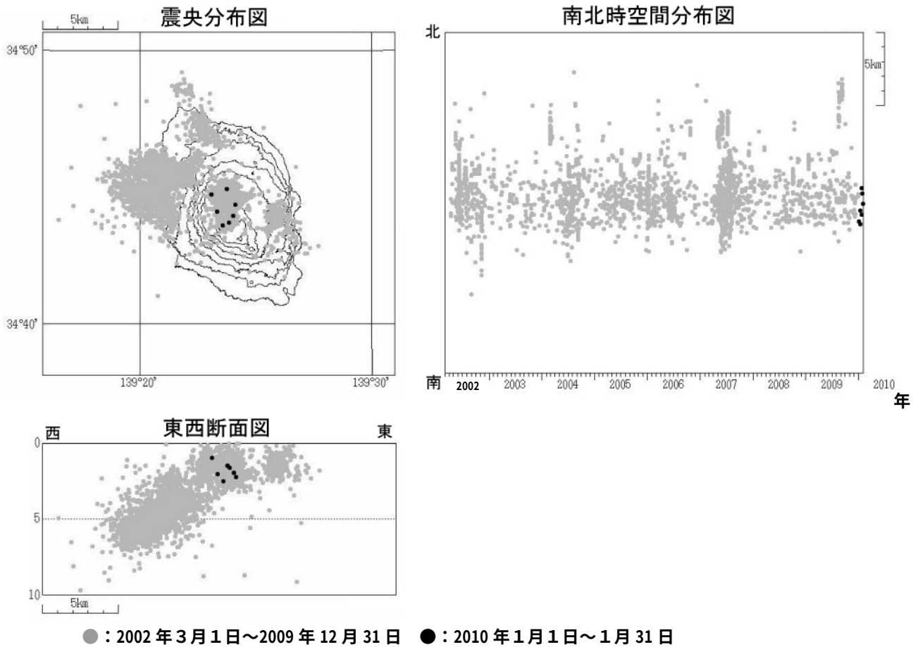
図 6 ※ 伊豆大島 震源分布図（2002 年 3 月 1 日～2010 年 1 月 31 日）
