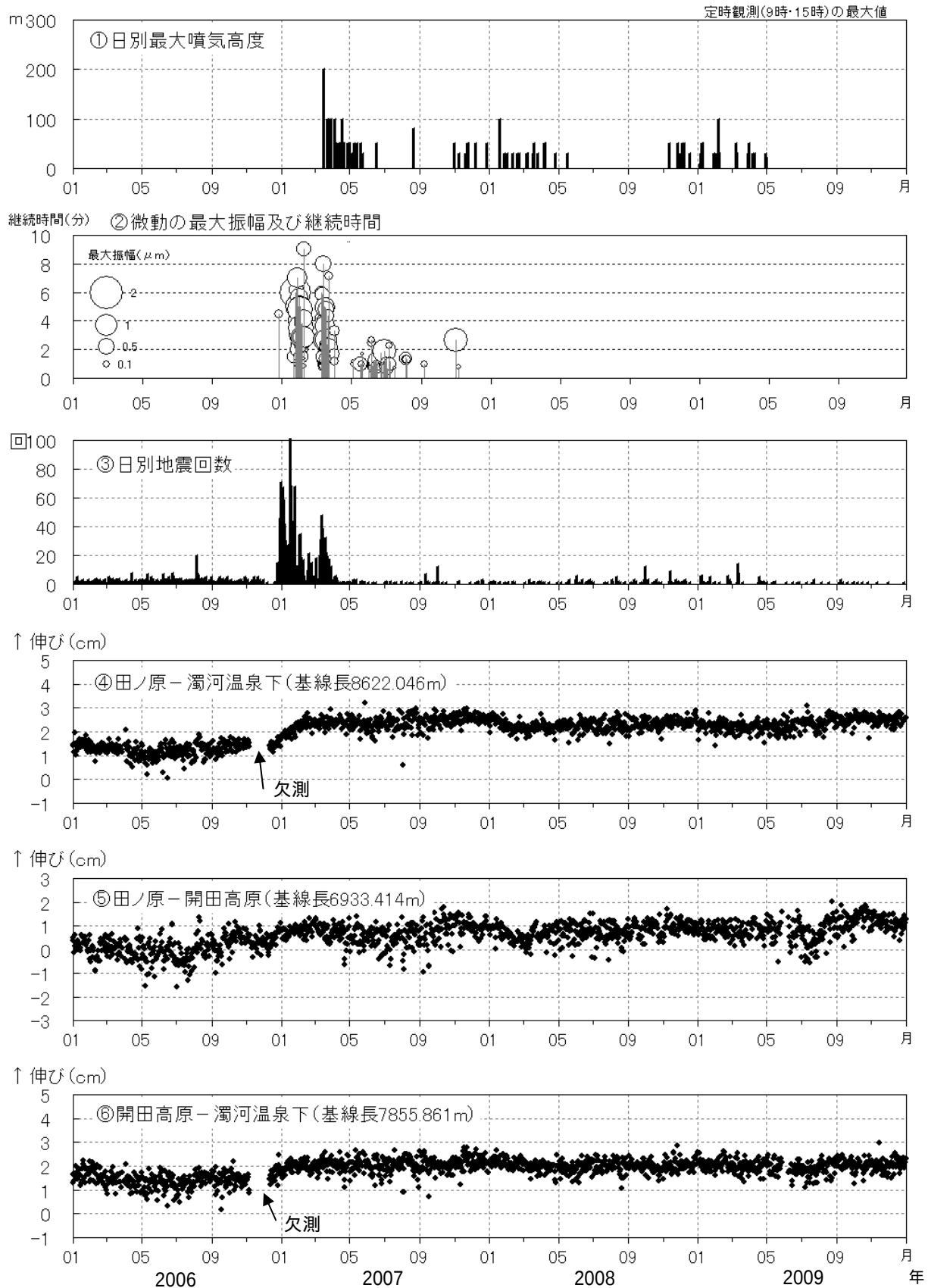
図2 御嶽山 最近の火山活動の推移（2006年1月1日～2009年12月31日）
