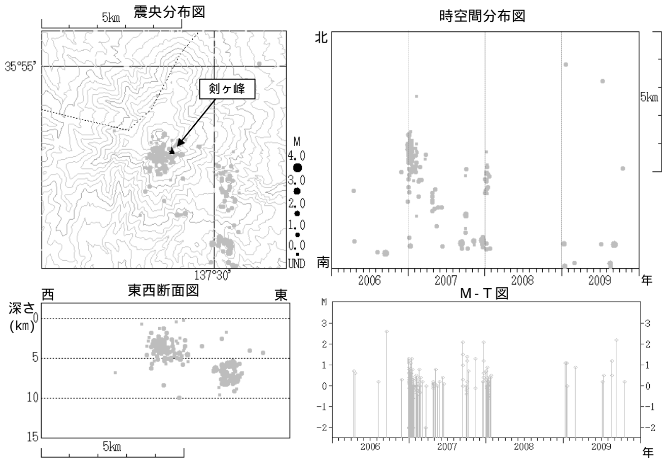
図3 御嶽山 震源分布図（2006年1月1日～2009年12月31日）
