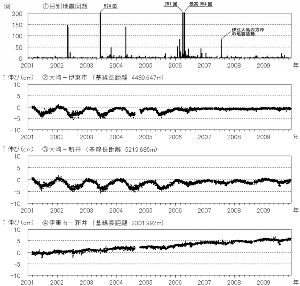
図2 伊豆東部火山群 最近の火山活動の推移（2001年1月～2009年11月）
