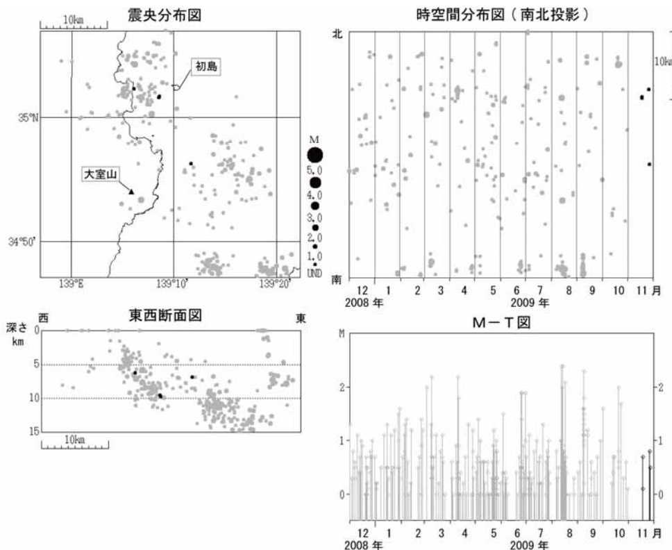
図 1 伊豆東部火山群 震源分布図（2008 年 12 月 1 日～2009 年 11 月 30 日）
