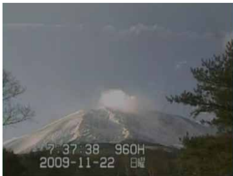
図 2 浅間山 山頂部の噴煙の状況 (11 月 22 日、鬼押し出しカメラによる)
