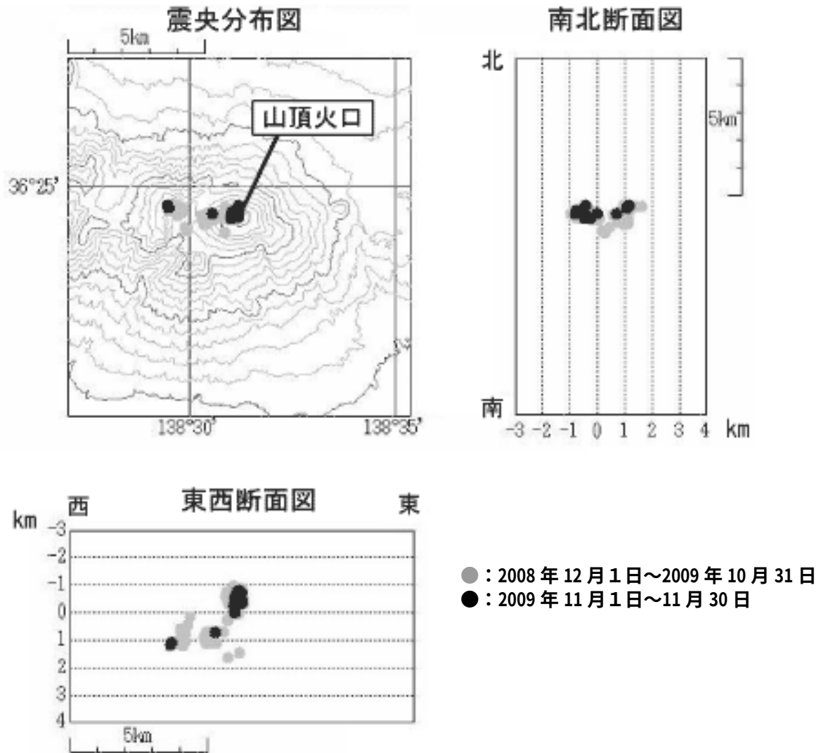
図 5 ※ 浅間山 震源分布図（2008 年 12 月 1 日～2009 年 11 月 30 日）
