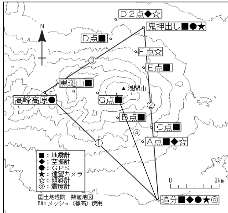
図 1 浅間山 気象庁の観測点配置図（小さな白丸は観測点位置を示しています） GPS 基線③は図 4 の⑨に、光波測距測線④は図 4 の⑩にそれぞれ対応しています。
