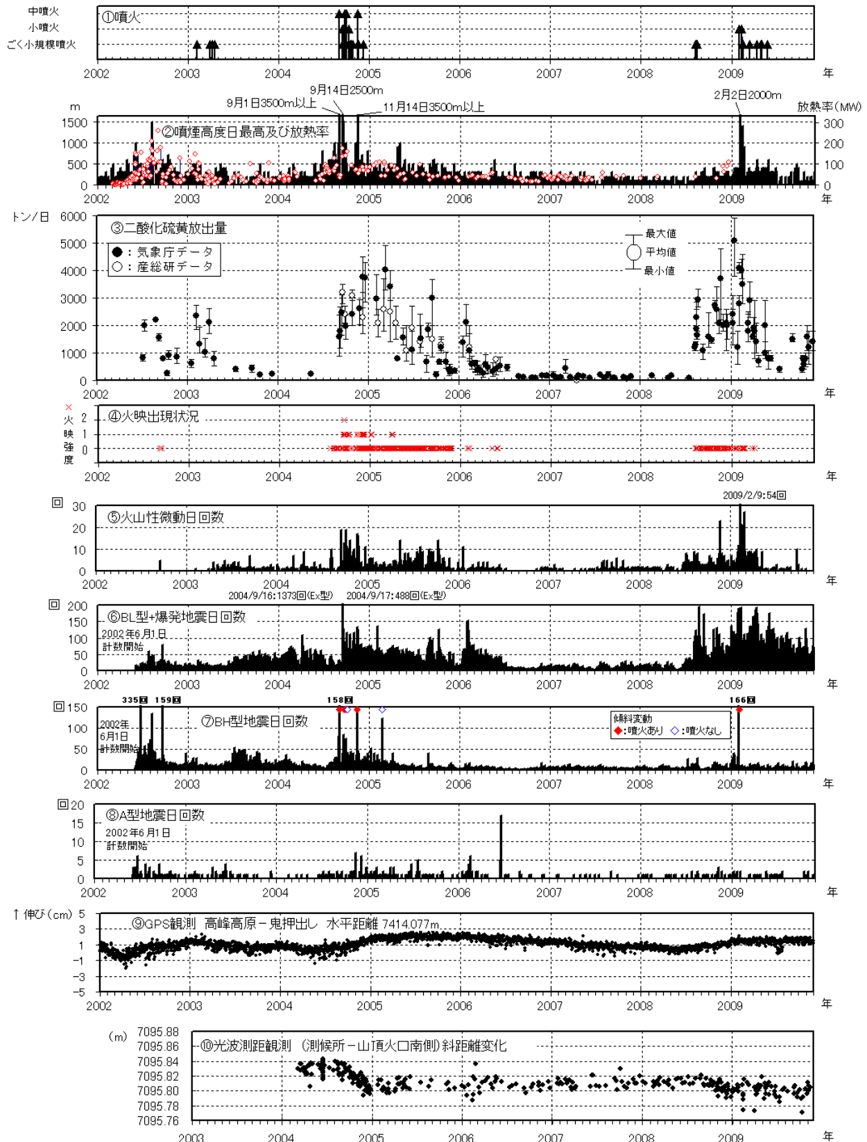
図 4 ※ 浅間山 最近の火山活動の推移 (2002 年 1 月 1 日～2009 年 11 月 30 日)
