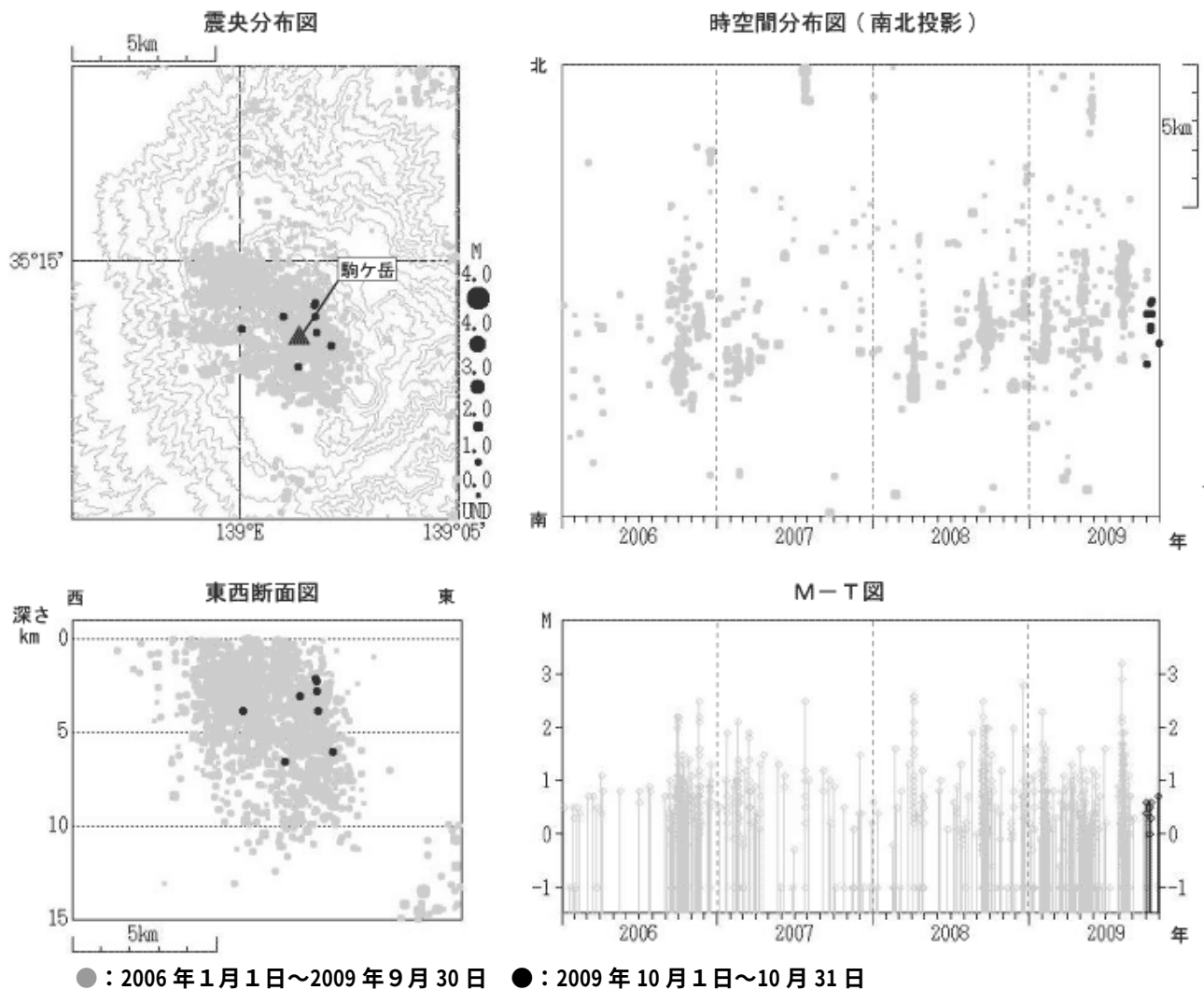
図 3 ※ 箱根山 震源分布図（2006 年 1 月 1 日～2009 年 10 月 31 日） M（マグニチュード）は地震の規模を表します。 図中の震源要素は一部暫定値が含まれており、後日変更することがあります。
