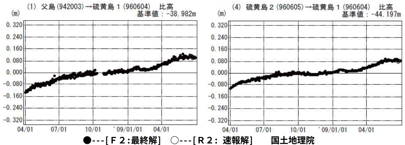
図1※ 硫黄島 国土地理院による GPS 観測結果 1) (2008 年 4 月 1 日～2009 年 6 月 30 日)
