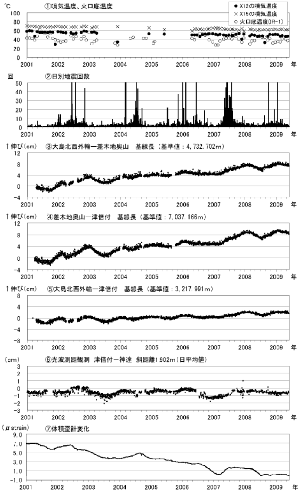
図5 伊豆大島 最近の火山活動経過図（2001年1月～2009年5月）
