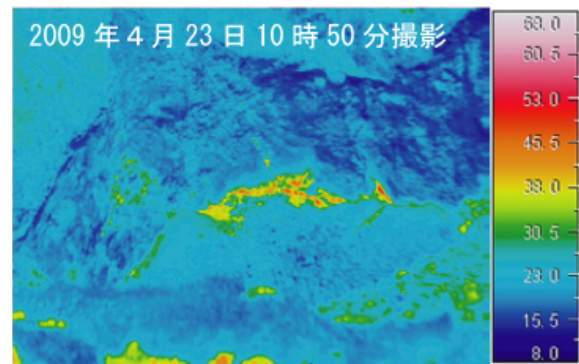
図1 伊豆大島 三原山山頂火口内及び山頂部の状況 右図の白円内は剣ガ峰付近のごく弱い噴気
