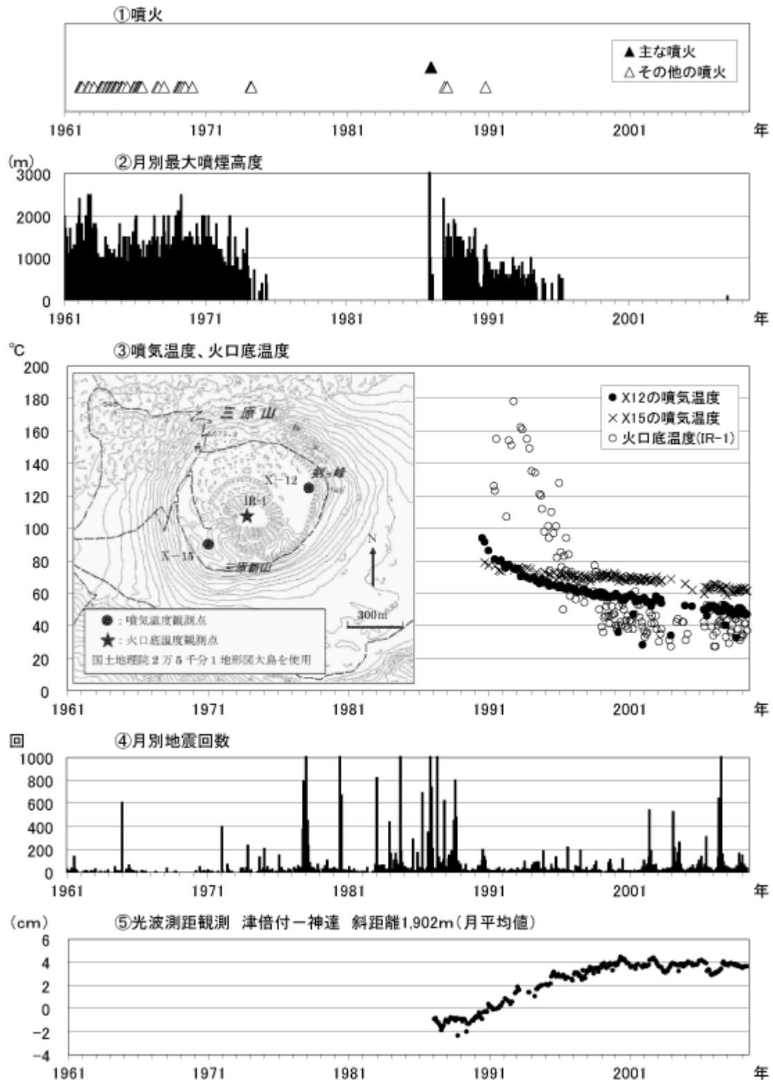
図4 伊豆大島 長期間の火山活動経過図（1961年1月～2009年5月）
