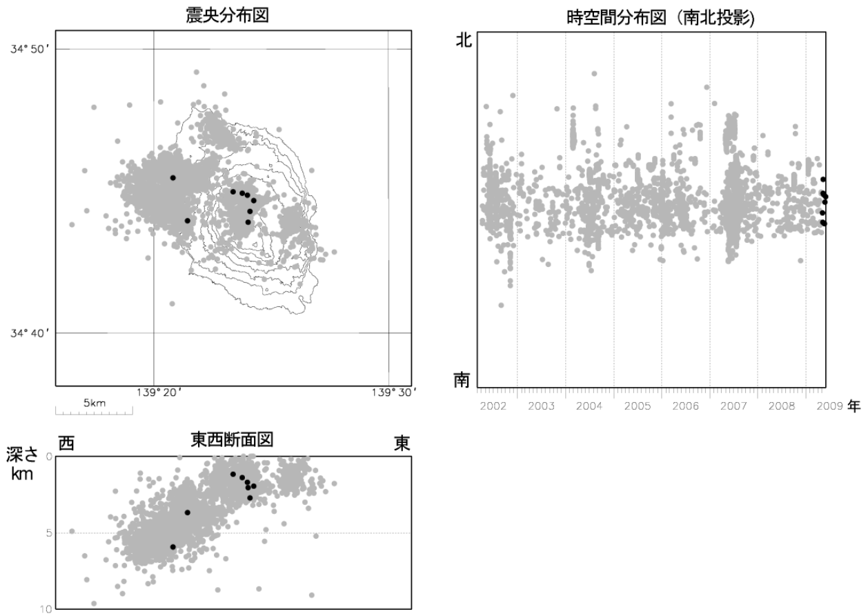
図 6 ※ 伊豆大島 震源分布図（2002 年 3 月 1 日～2009 年 5 月 31 日）
