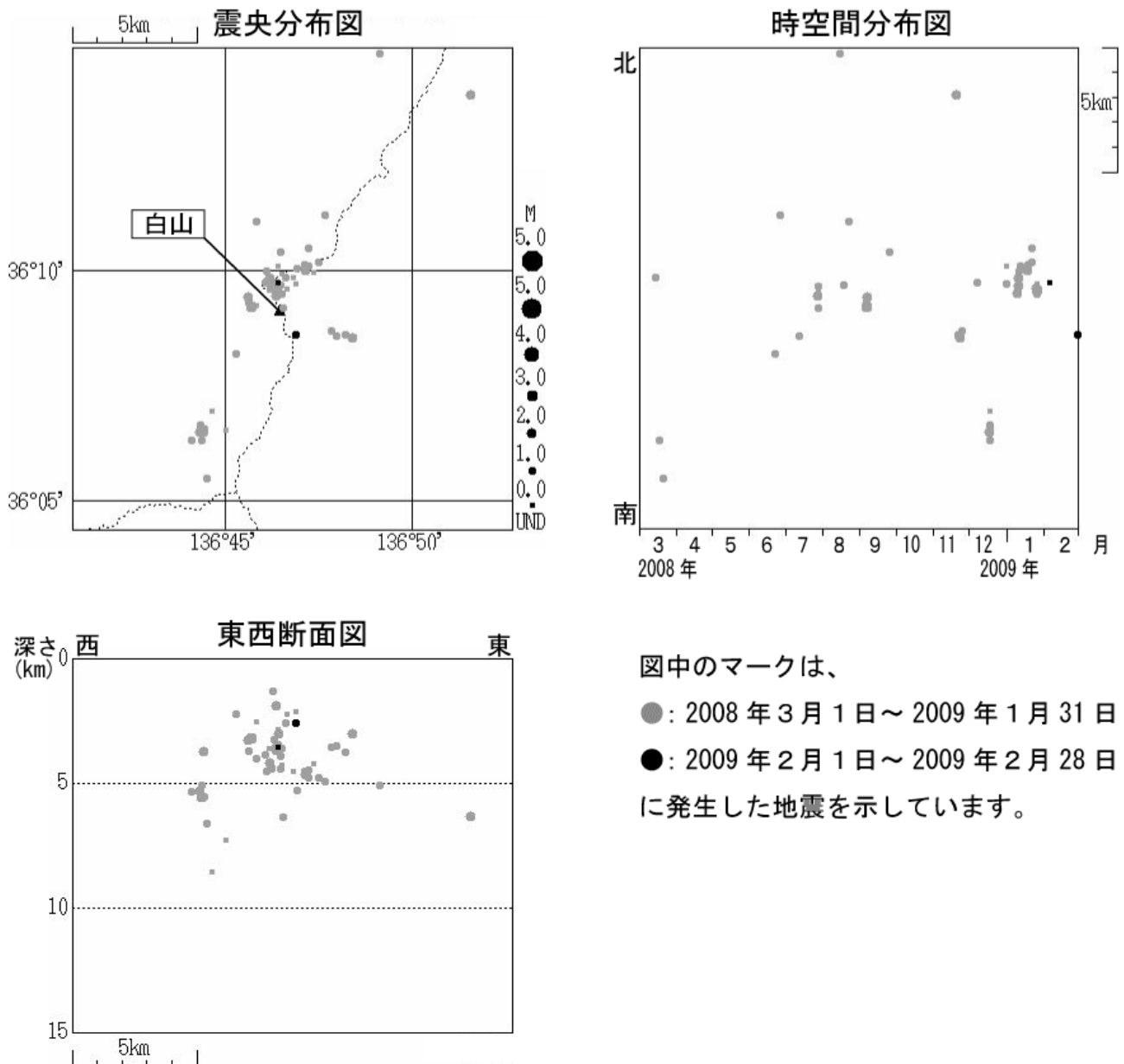
図3※ 白山 震源分布図（2008年3月1日～2009年2月28日）
