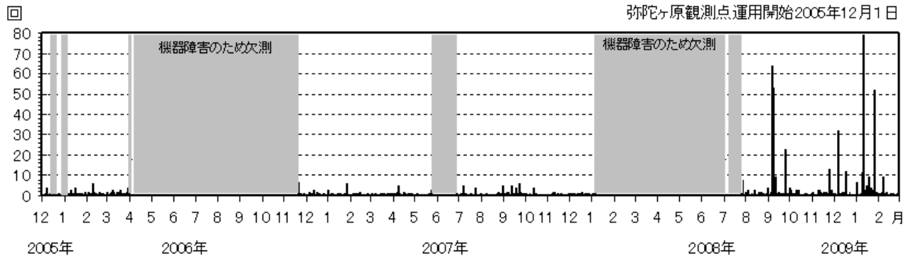
図2 白山 日別地震回数（2005年12月1日～2009年2月28日）
