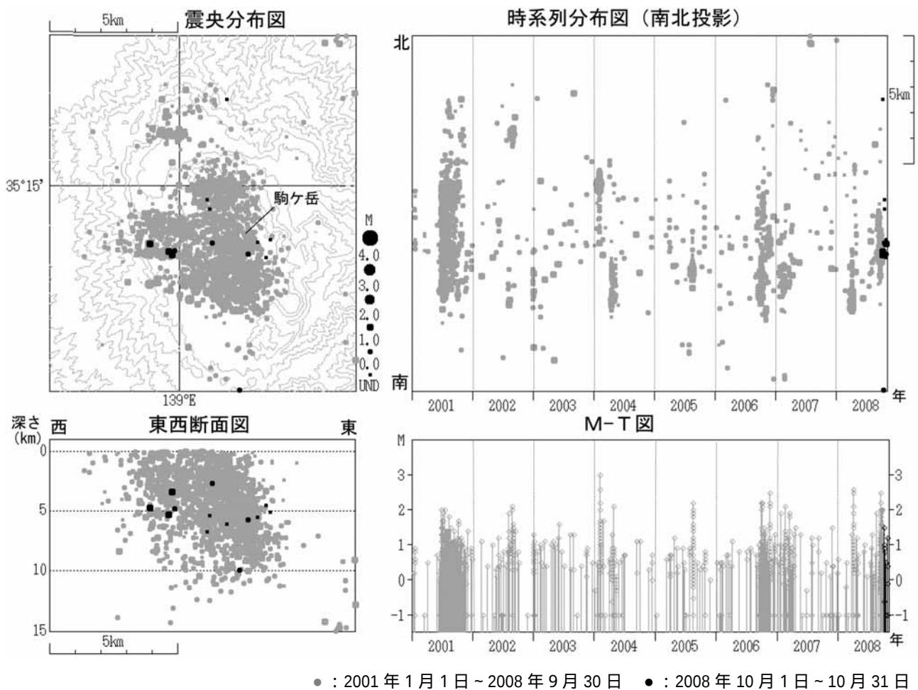
図3 箱根山 震源分布図（2001 年 1 月 1 日～2008 年 10 月 31 日）
