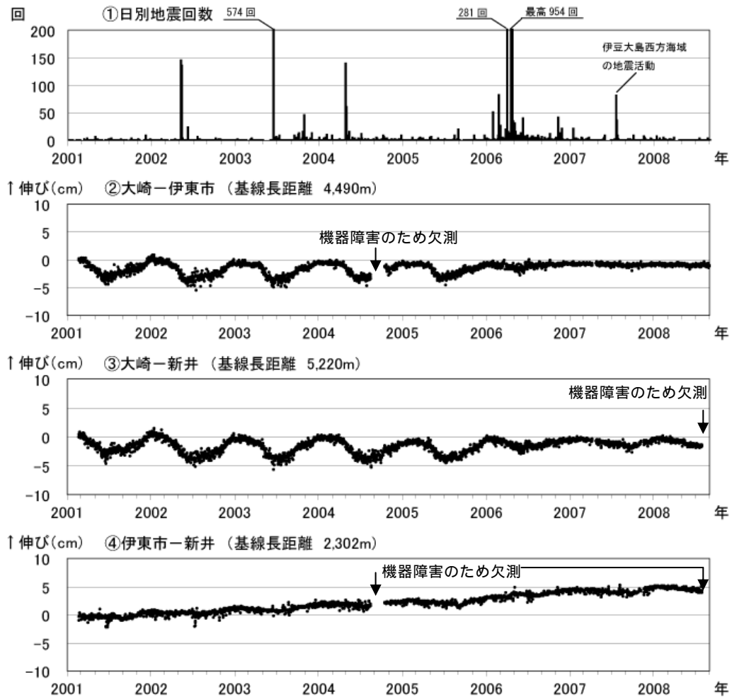
図2 伊豆東部火山群 最近の火山活動の推移（2001年1月～2008年8月）
