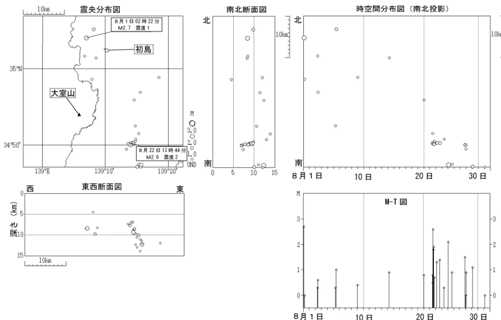
図 1 伊豆東部火山群 地震活動経過図（2008 年 8 月 1 日～8 月 31 日）
