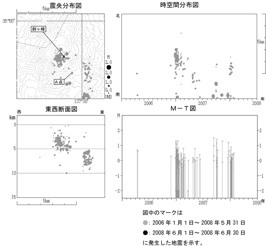
図 4 ※ 御嶽山 山頂付近の地震活動（2006 年 1 月 1 日～2008 年 6 月 30 日） 今期間発生した地震のうち震源が求まったものを表示しています。 +印は気象庁地震観測点（A 点）の位置を示しています。M（マグニチュード）は地震の規模を表します。図中の震源要素は一部暫定値で、後日変更することがあります。
