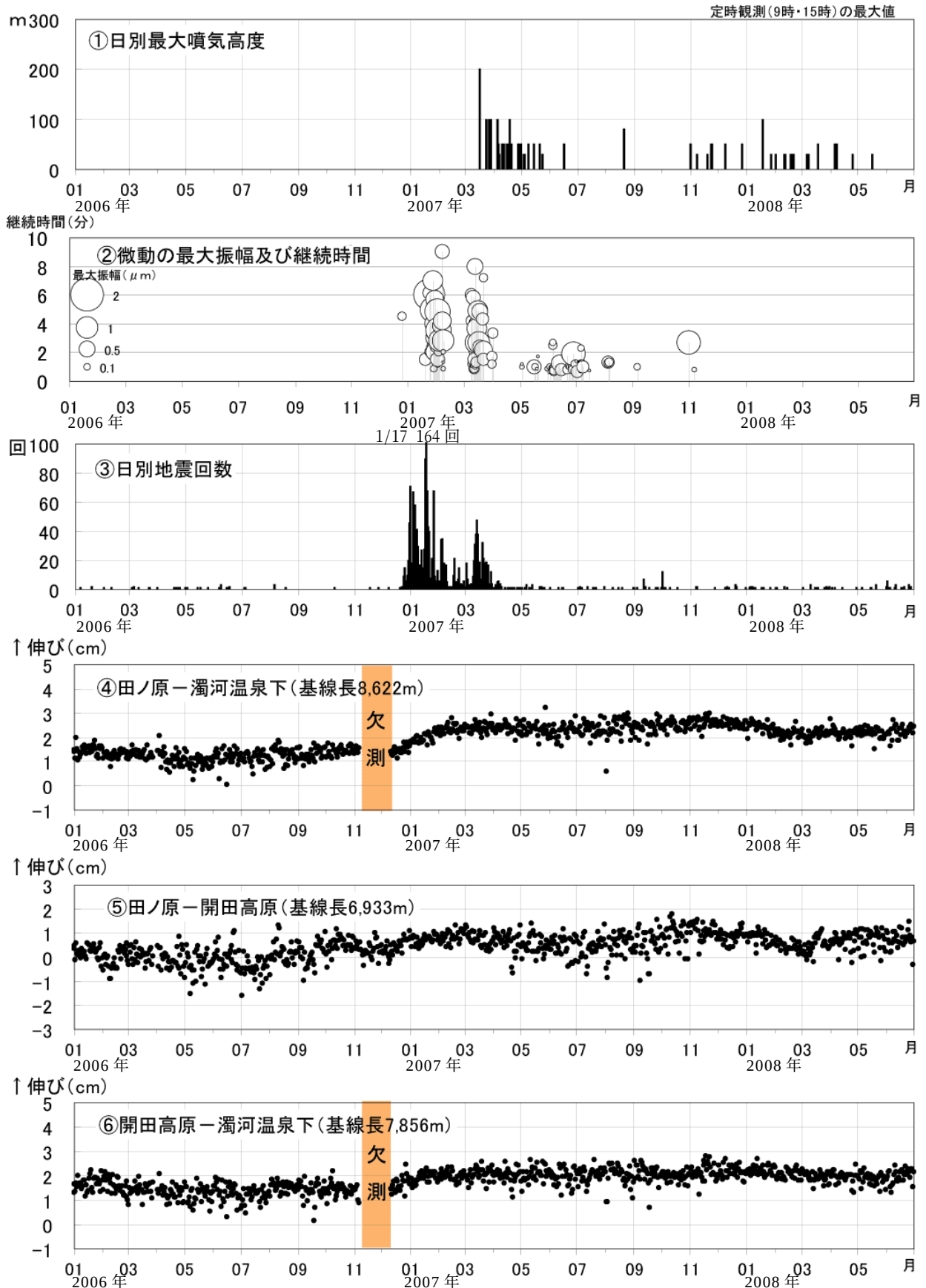
図2 御嶽山 最近の火山活動の推移（2006年1月1日～2008年6月30日）
