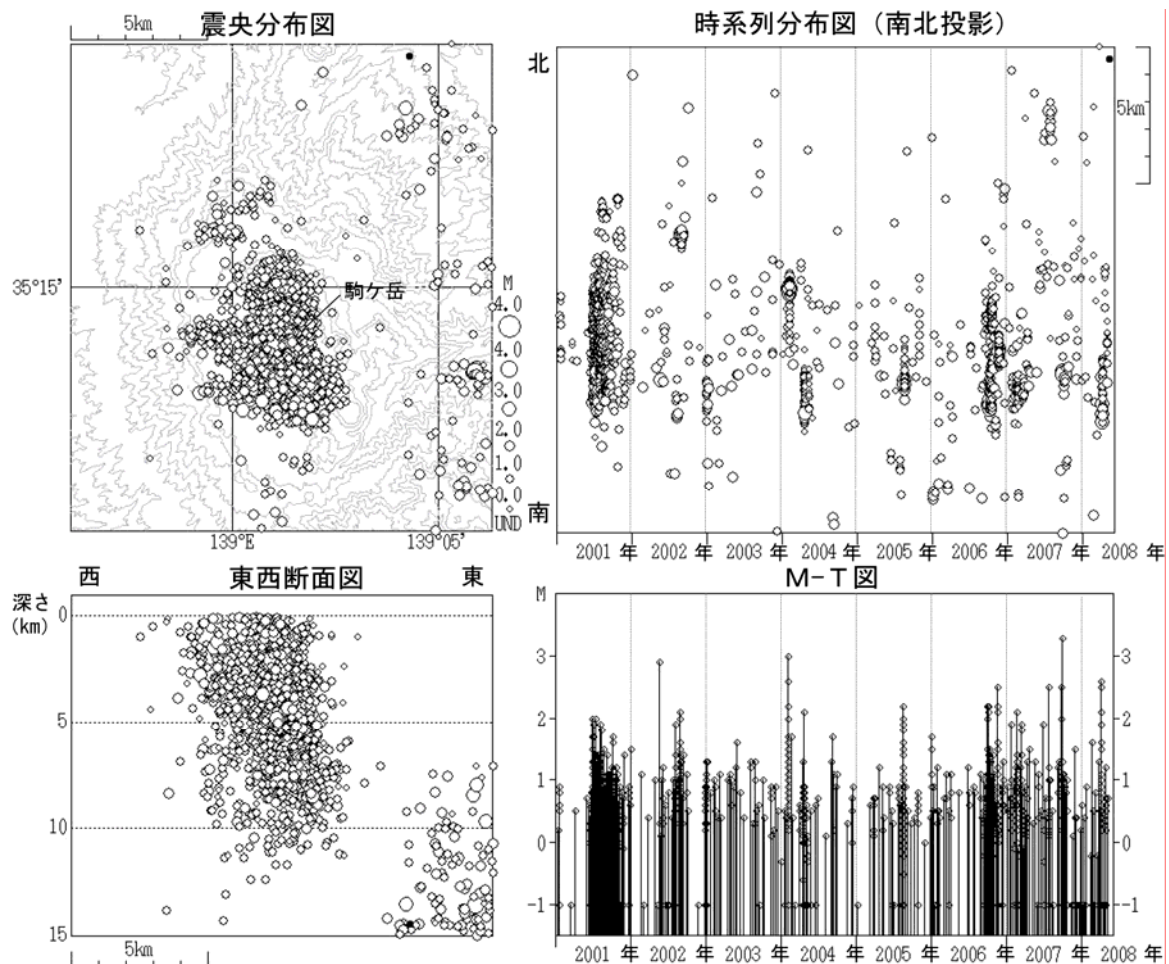
図 2 箱根山 地震活動経過（2001年1月1日～2008年5月31日）
