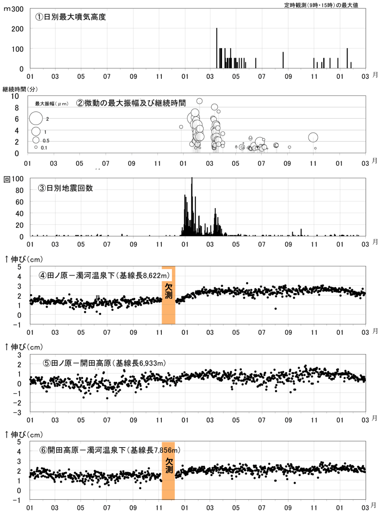
図2 御嶽山 最近の火山活動の推移（2006年1月1日～2008年2月29日）
