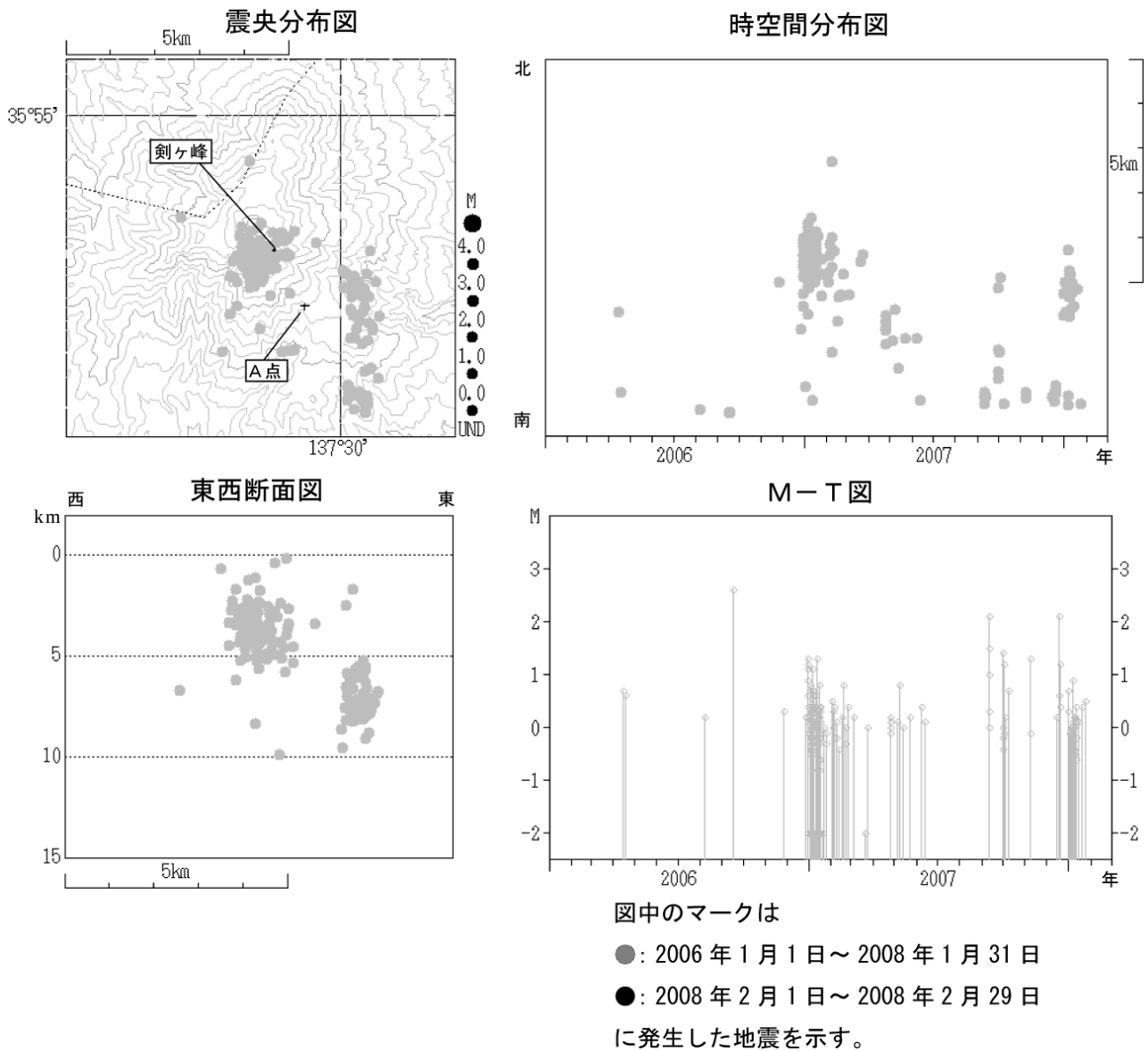
図 3 ※ 御嶽山 山頂付近の地震活動（2006 年 1 月 1 日～2008 年 2 月 29 日） +印は気象庁地震観測点（A 点）の位置を示しています。M（マグニチュード）は地震の規模を表します。図中の震源要素は一部暫定値で、後日変更することがあります。
