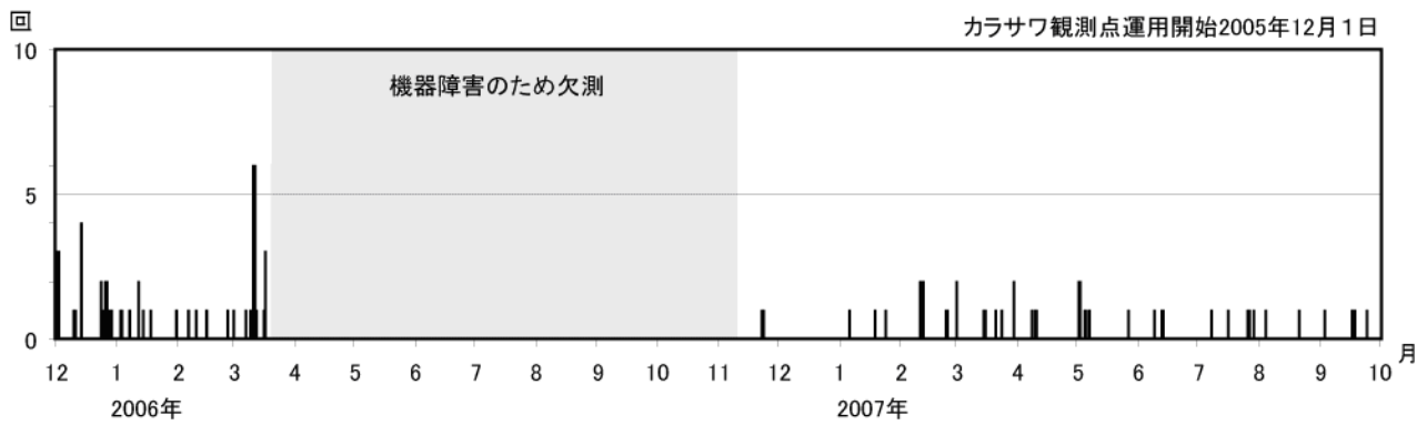
図2 新潟焼山 日別地震回数（2005年12月1日～2007年9月30日）
