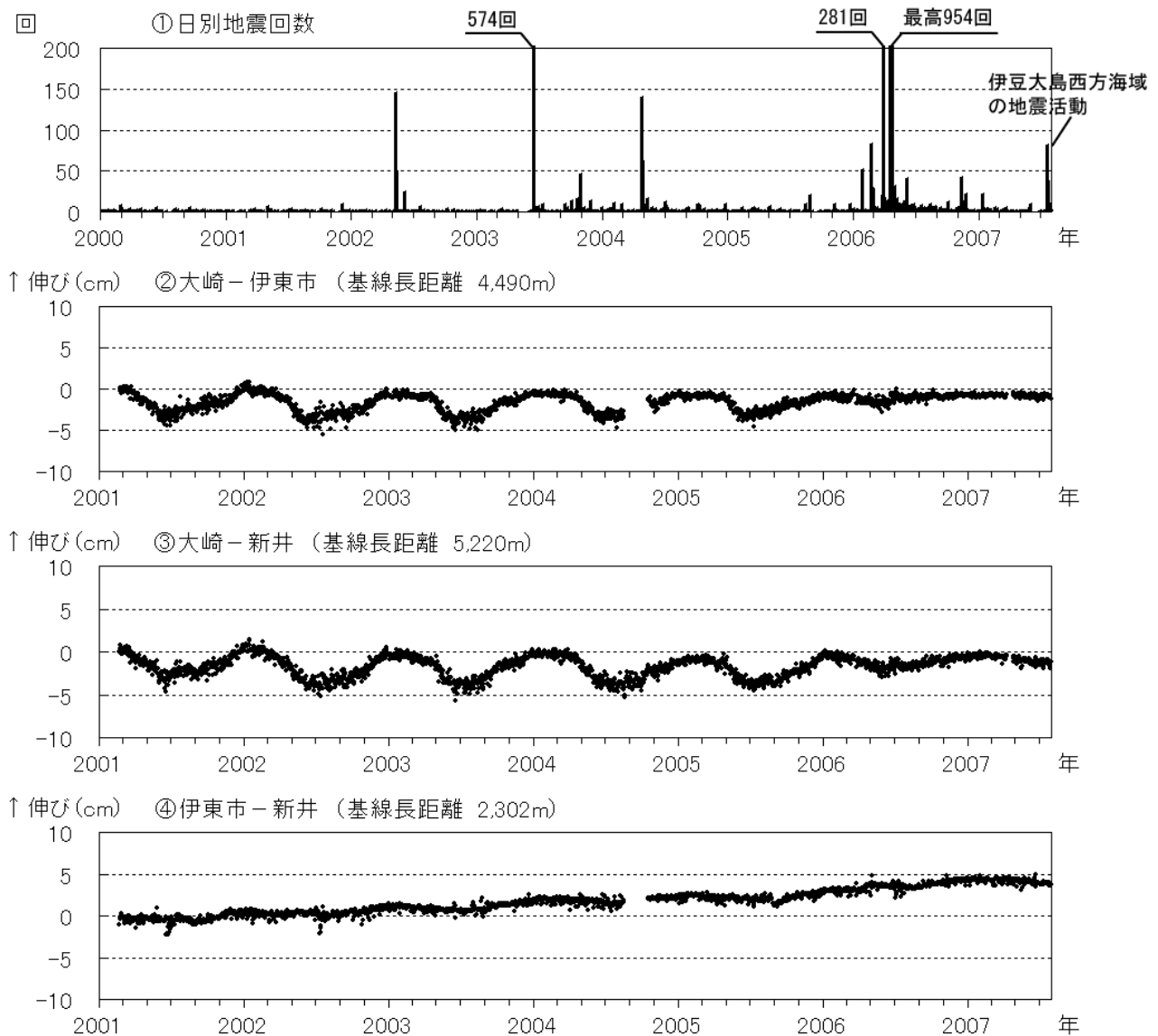
図2 伊豆東部火山群 最近の火山活動の推移 (2001年1月～2007年7月)
