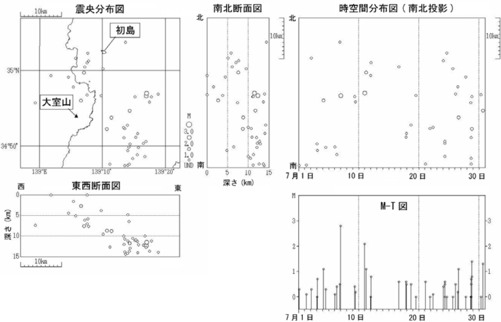
図1※ 伊豆東部火山群 地震活動経過図（2007 年 7 月 1 日～7 月 31 日）
