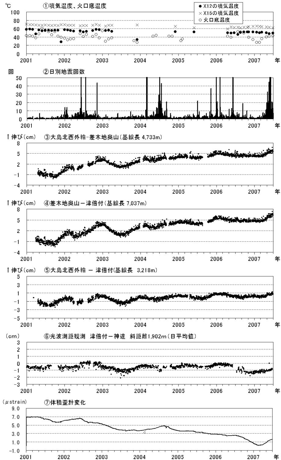
図 5 伊豆大島 最近の火山活動経過図（2001 年 1 月～2007 年 6 月）
