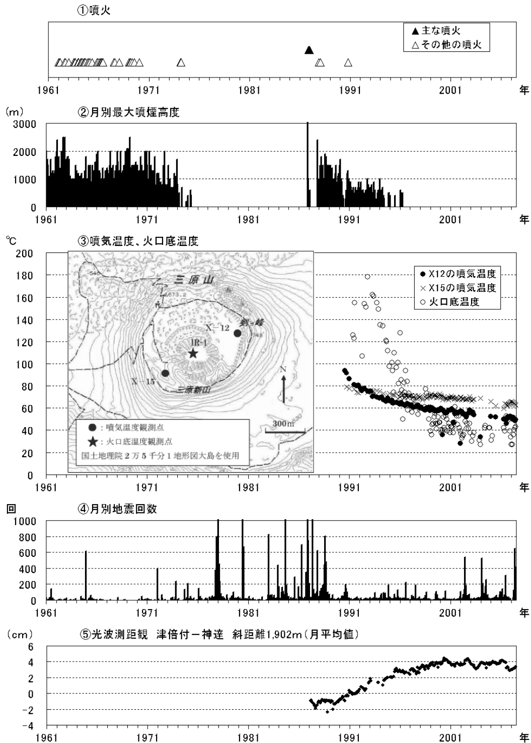
図 4 伊豆大島 長期間の火山活動経過図（1961 年 1 月～2007 年 6 月）
