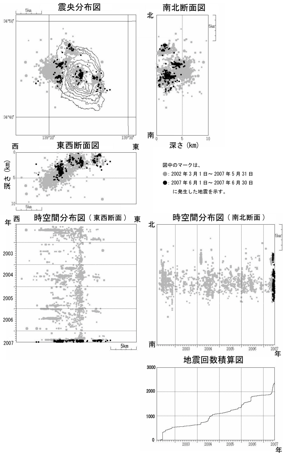
図 6 伊豆大島 震源分布図（2002 年 3 月 1 日～2007 年 6 月 30 日）
