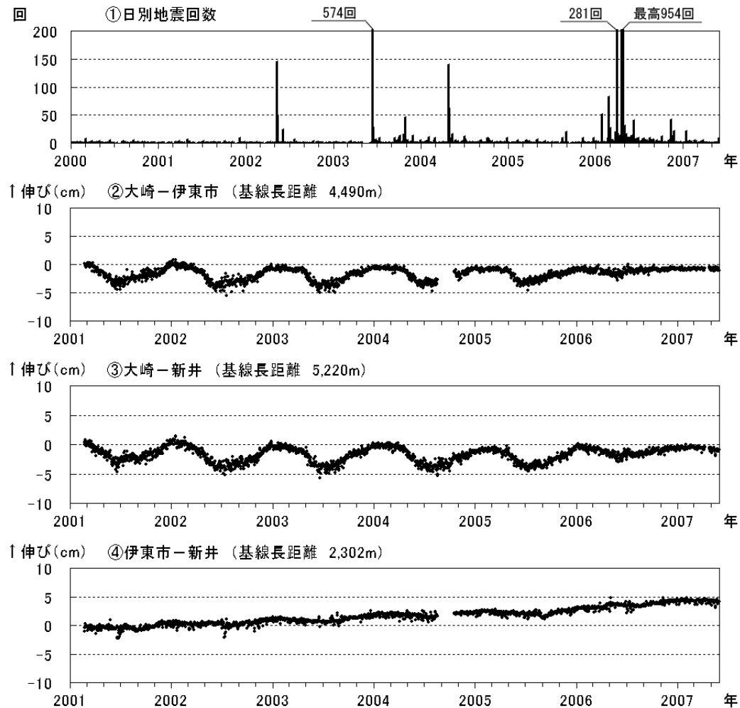
図2 伊豆東部火山群 最近の火山活動の推移（2001年1月～2007年5月）
