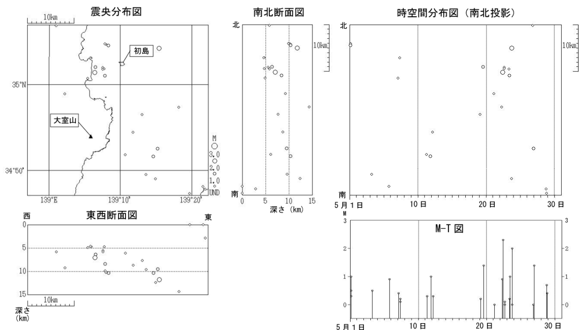
図1※ 伊豆東部火山群 地震活動経過図（2007年5月1日～5月31日）
