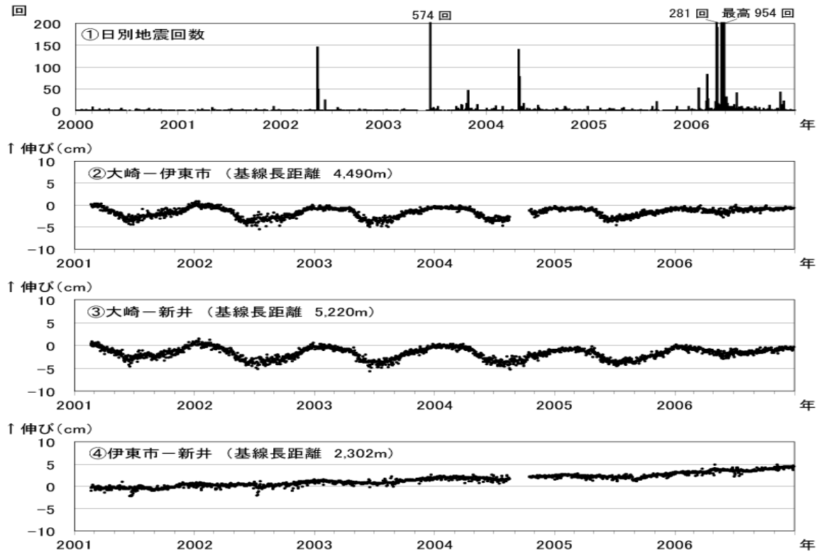
図2 伊豆東部火山群 最近の火山活動の推移（2001 年 1 月～2006 年 12 月）
