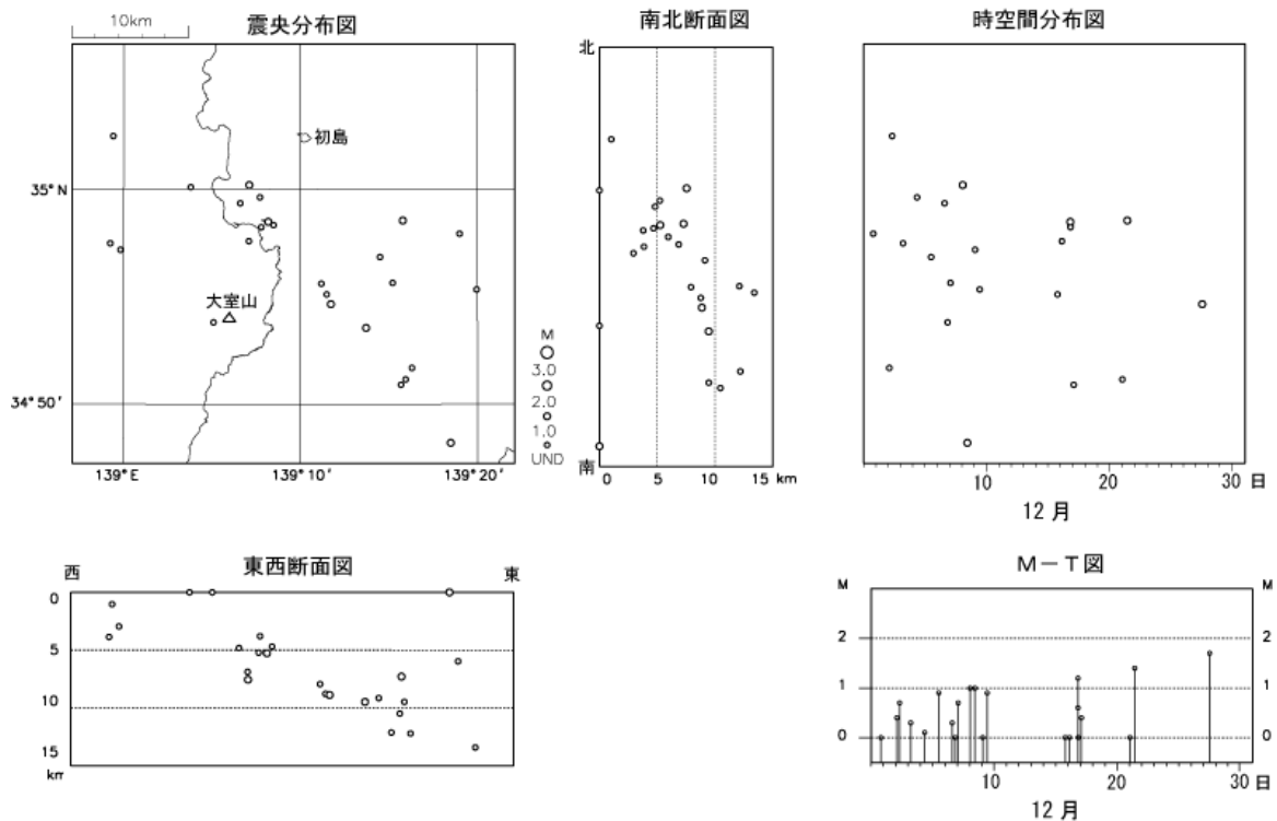
図 1 ※ 伊豆東部火山群 地震活動経過図（2006 年 12 月 1 日～12 月 31 日）
