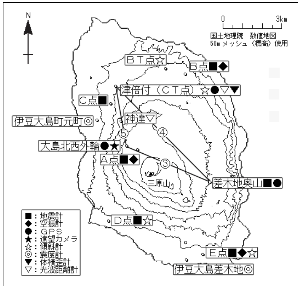
図9 伊豆大島 気象庁の観測点配置図（小さな白丸は観測点位置を示しています） GPS 基線③～⑤は図6の③～⑤に対応しています。
