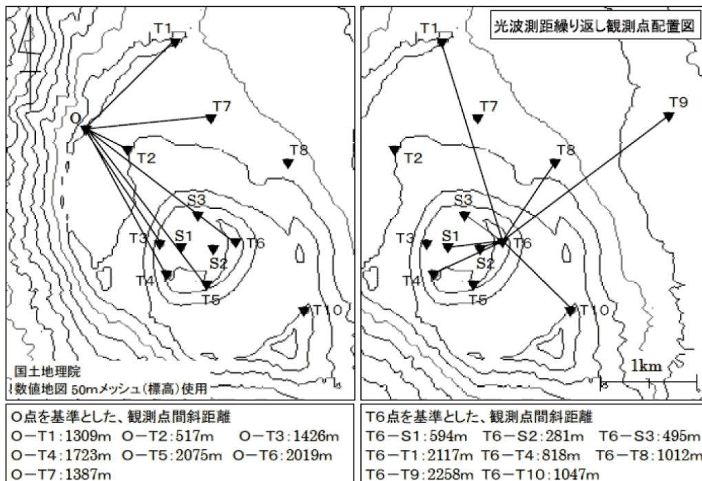
図 8 伊豆大島 光波距離計繰り返し観測点の配置図
