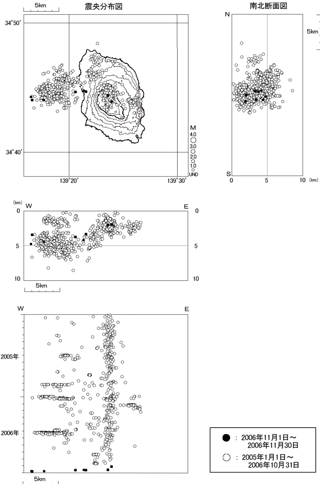
図 4 伊豆大島 震源分布図（2005 年 1 月 1 日～2006 年 11 月 30 日）
