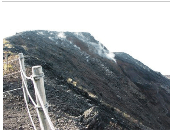
図 2 伊豆大島 三原新山の噴気の状況（2006 年 11 月 29 日、火口縁から撮影）
