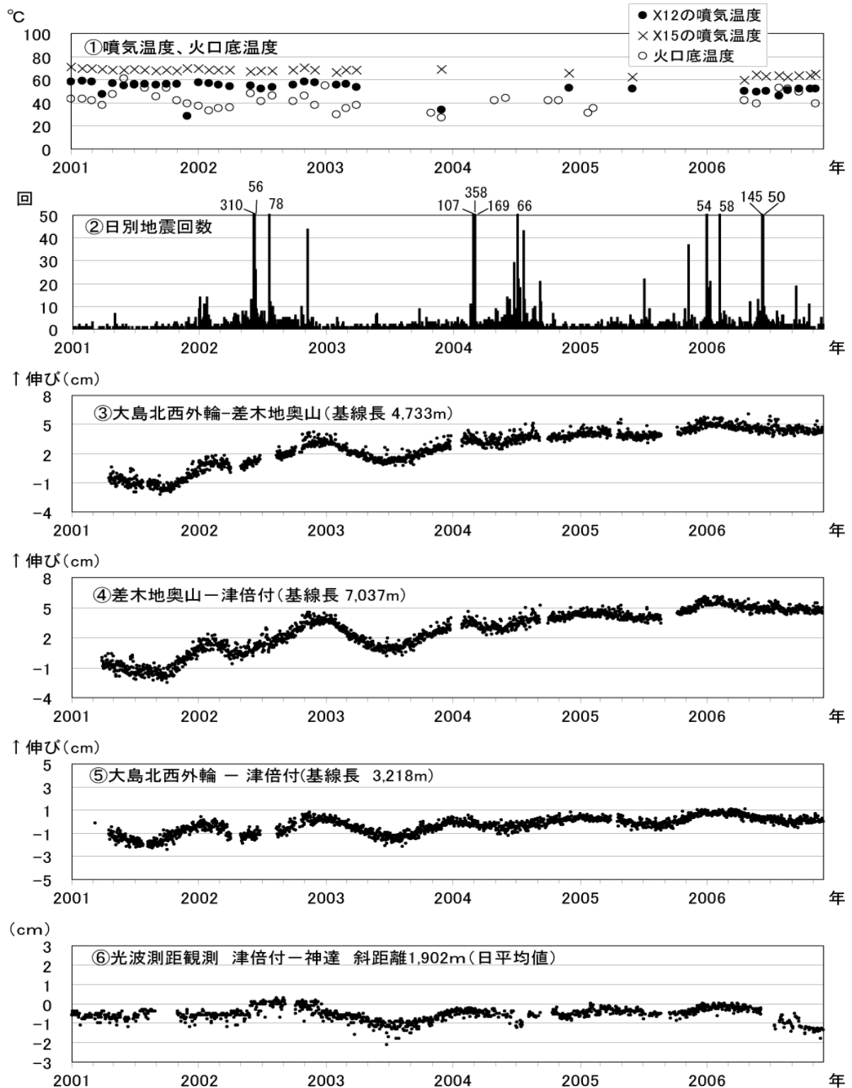
図 6 伊豆大島 最近の火山活動経過図（2001 年 1 月～2006 年 11 月）
