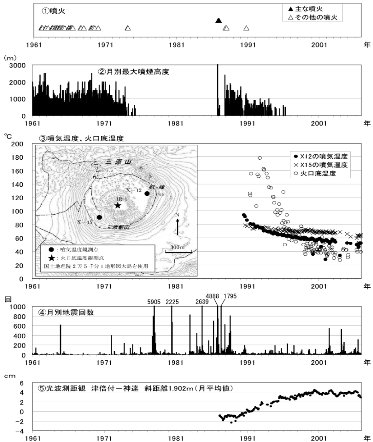
図5 伊豆大島 長期間の火山活動経過図（1961 年 1 月～2006 年 11 月）
