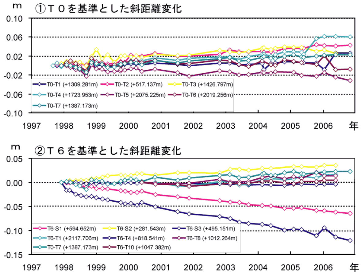
図 7 伊豆大島 光波距離計の観測による斜距離変化（1997 年 12 月～2006 年 11 月）
