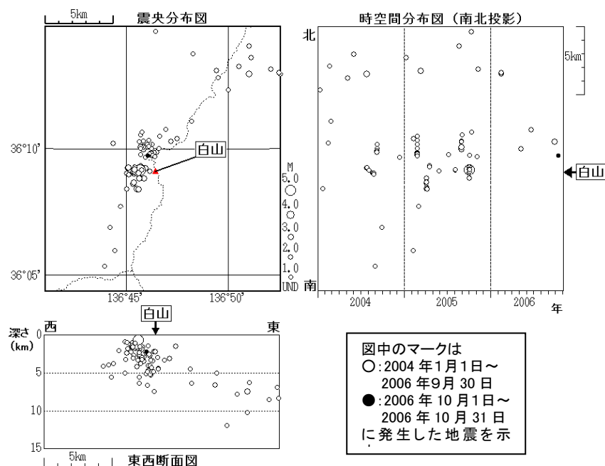
図 1 ※ 白山 山体及びその周辺の地震活動（2004 年 1 月 1 日～2006 年 10 月 31 日）
