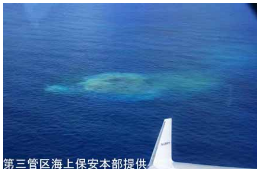
図 1 福德岡ノ場 変色水の状況（9 月 13 日）
