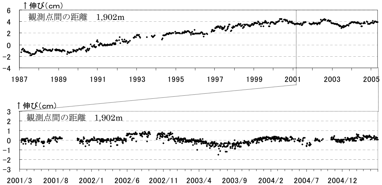
図4 伊豆大島 光波距離計（津倍付～神達）斜距離変化 上：旬平均値（1987 年 1 月～2005 年 4 月） 下：日平均値（2001 年 3 月 1 日～2005 年 4 月 30 日）
