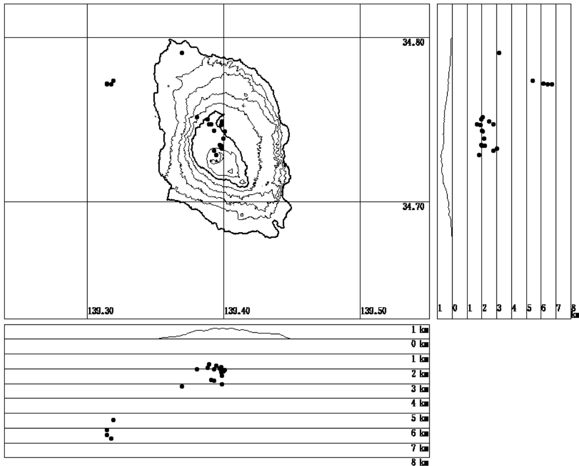
図 2 伊豆大島 2005 年 4 月の地震活動
