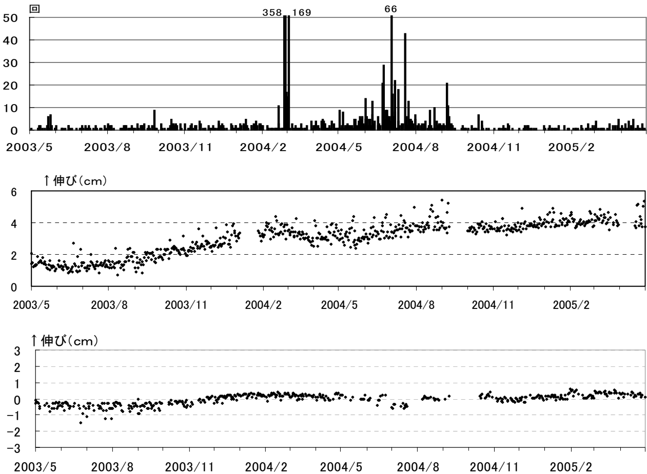
図5 伊豆大島 最近2年間（2003 年 5 月～2005 年 4 月）の活動 上：地震回数 中：①大島北西外輪～差木地奥山 GPS 観測 下：光波距離計（津倍付～神達）観測
