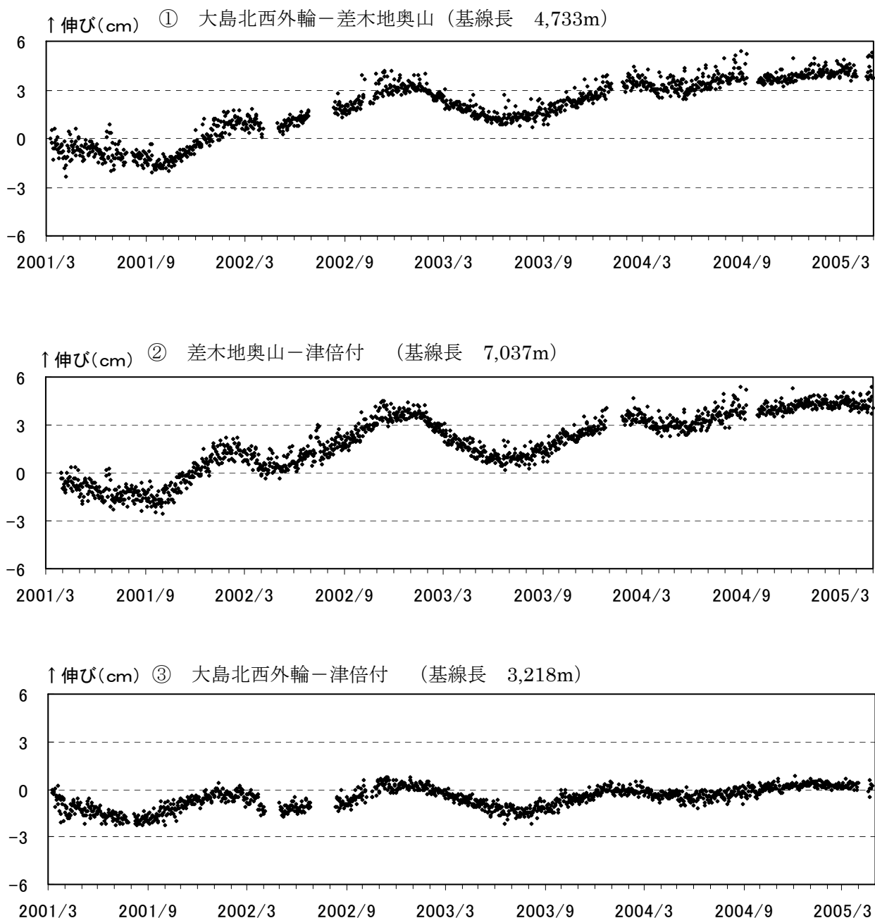
図 3 伊豆大島 GPS 観測結果（基線長変化）（2001 年 3 月 7 日～2005 年 4 月 30 日）
