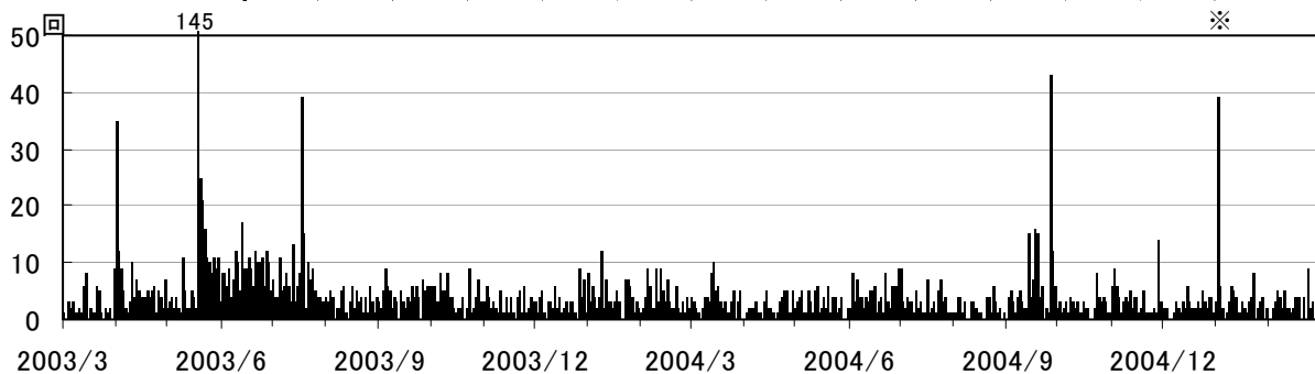
図 1 御嶽山 火山性地震日別回数（2003 年 3 月 1 日～2005 年 2 月 28 日）
