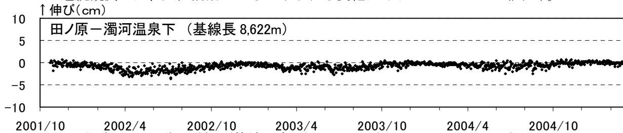
図 2 御嶽山 GPS 観測結果(基線長変化)（2001 年 10 月 23 日～2005 年 2 月 28 日）
