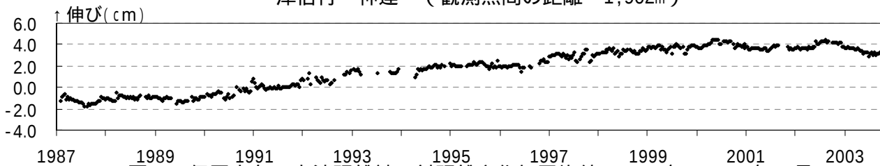
図5 伊豆大島 光波距離計 斜距離変化旬平均値(1987年~2003年8月) 津倍付 - 神達 (観測点間の距離 1,902m)
