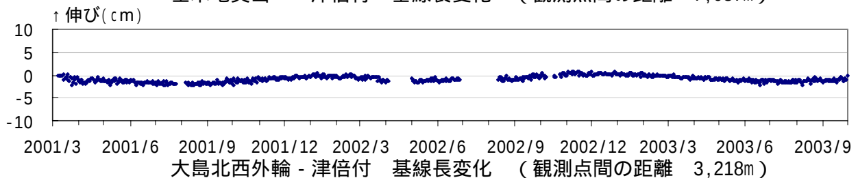
図3 伊豆大島 GPS観測結果(2001年3月7日~2003年9月30日)
