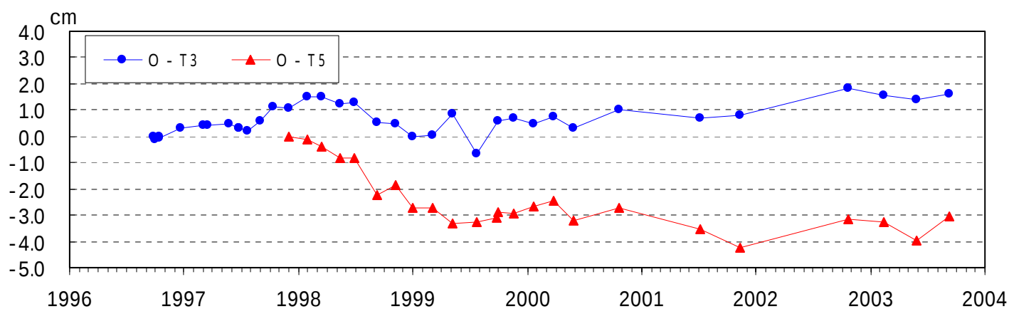
図6 伊豆大島 光波距離計 O点を基準とした斜距離変化 (1996年9月～2003年9月)
