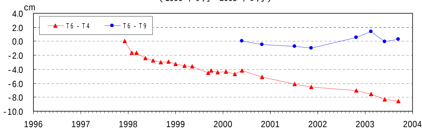
図7 伊豆大島 光波距離計 T6点を基準とした斜距離変化 (1997年12月～2003年9月)
