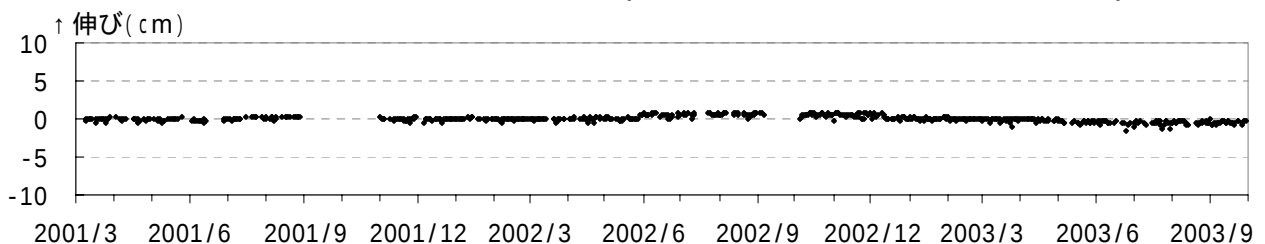
図4 伊豆大島 光波距離計 斜距離変化日平均値(2001年3月1日~2003年8月31日) 津倍付 - 神達 (観測点間の距離 1,902m)
