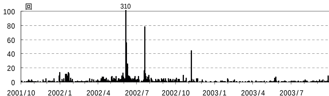
図1 伊豆大島 火山性地震日別回数(2001 年 10 月 1 日 ~ 2003 年 9 月 30 日)
