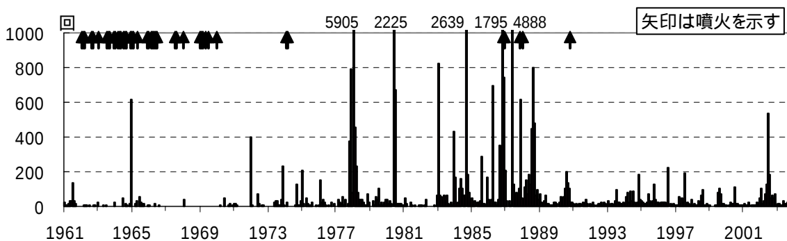
図2 伊豆大島 火山性地震月別回数(1961 年 1 月 ~ 2003 年 9 月)
