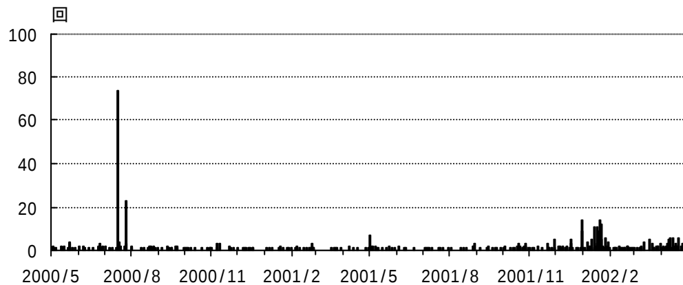
伊豆大島 火山性地震日別回数(2000年 5月～2002年 4月)
