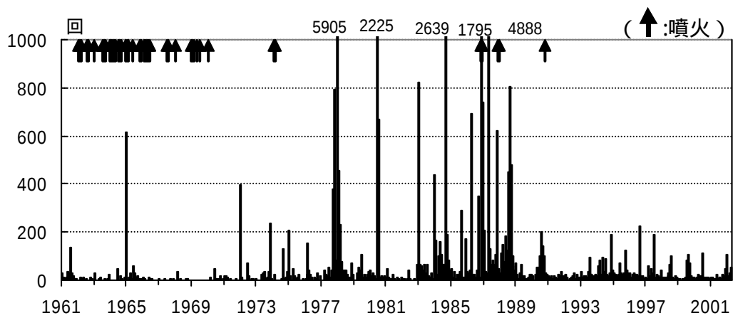
伊豆大島 火山性地震月別回数(1961年 1月～2002年 4月)
