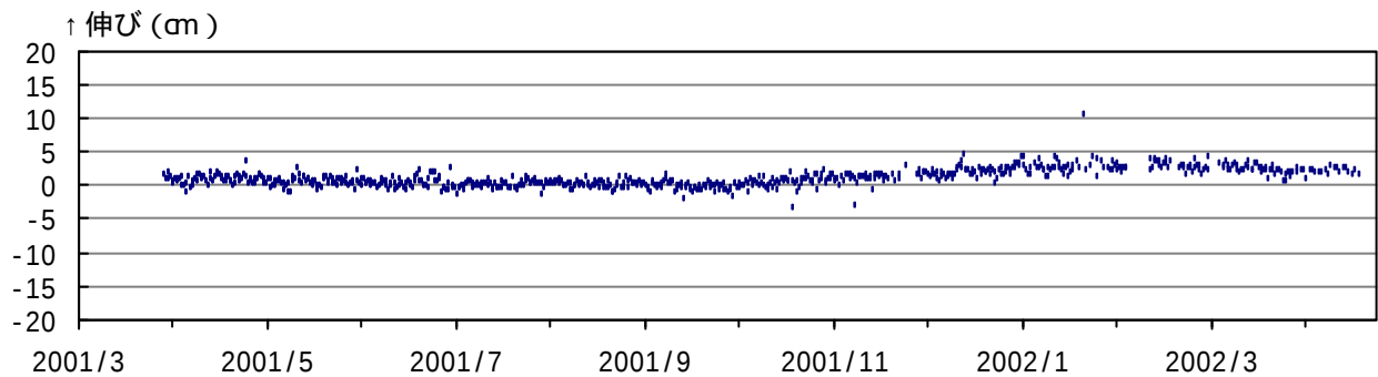
伊豆大島 GPS観測結果 (2001年 3月 1日～2002年 4月30日) 差木地検査網 - 旧測候所跡地 基線長
