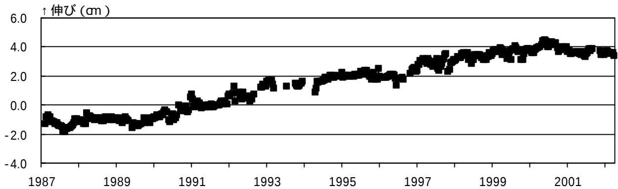
伊豆大島 光波距離計 斜距離勾平均値 (1987年～2002年 4月)
