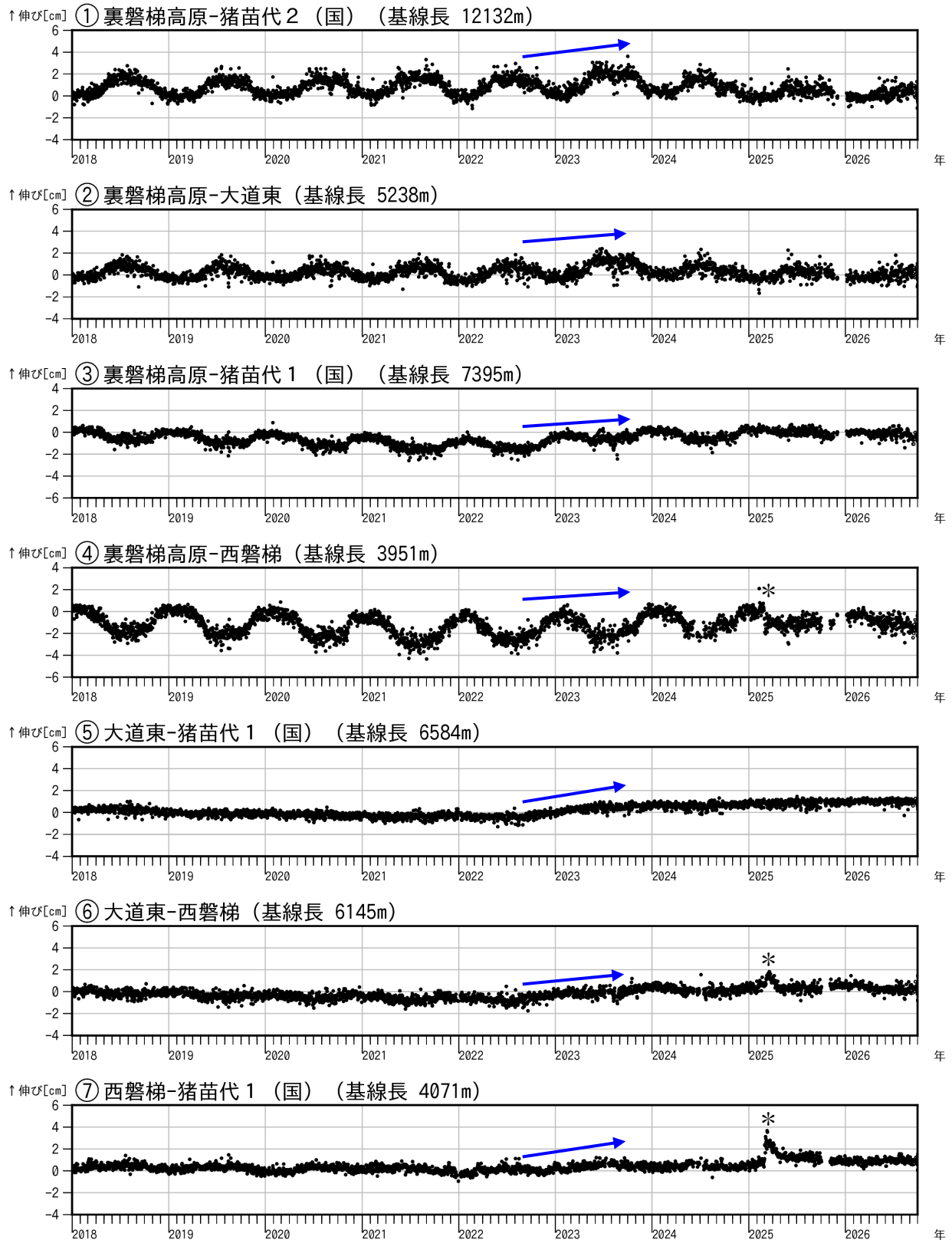
図6 磐梯山 GNSS 基線長変化図（2018年1月～2026年9月）
