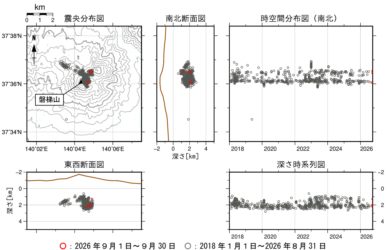
図 5 磐梯山 震源分布図（2018 年 1 月～2026 年 9 月）
