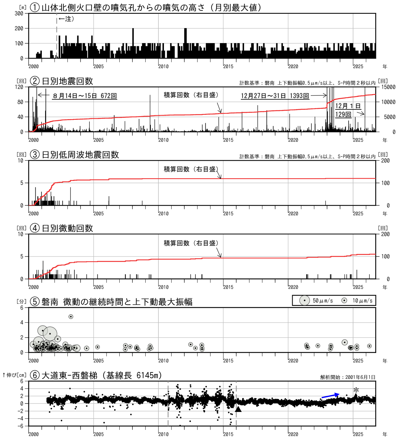
図3 磐梯山 火山活動経過図（2000年1月～2026年9月）
