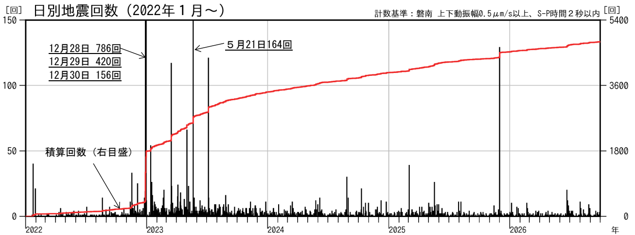
図 4 磐梯山 地震回数（2022 年 1 月～2026 年 9 月）
