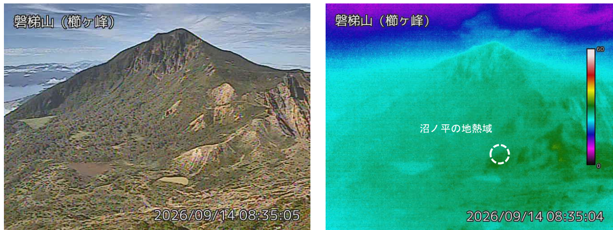
図2 磐梯山 沼ノ平周辺の状況と地表面温度分布（9月14日）
