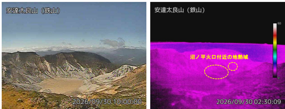
図2 安達太良山 沼ノ平火口周辺の状況と地表面温度分布の状況（9月30日）
