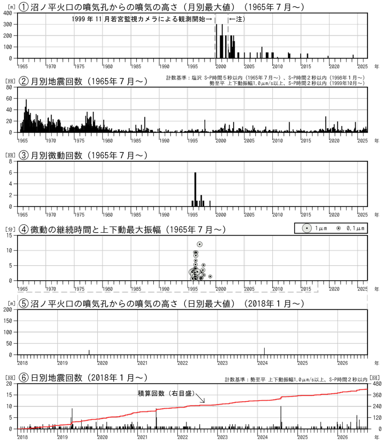
図3 安達太良山 火山活動経過図（1965年7月～2026年9月）
