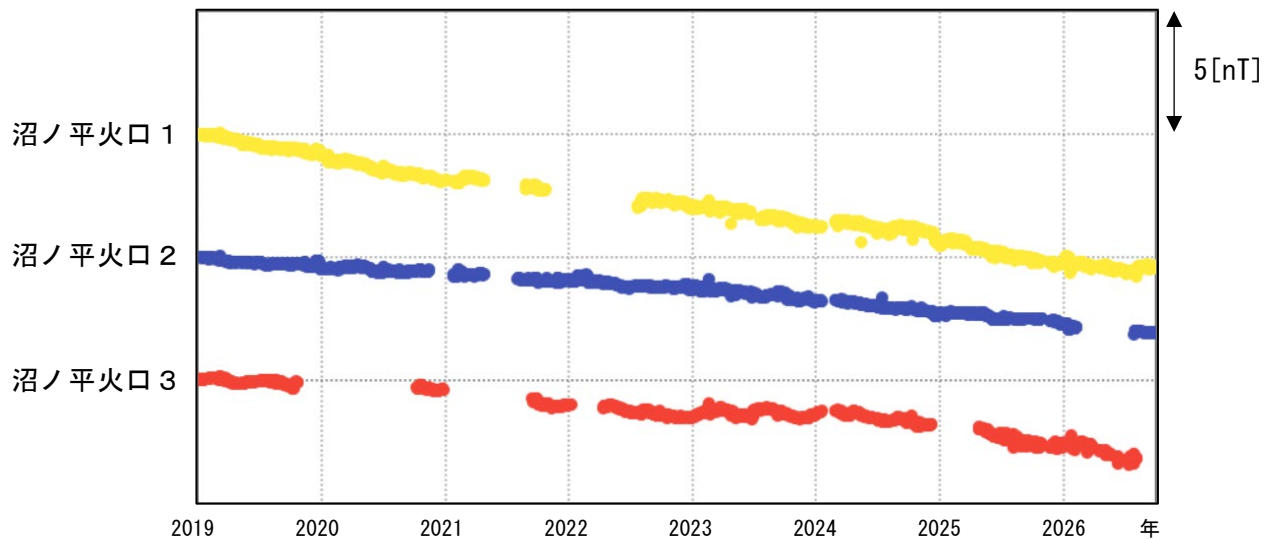
図5 安達太良山 全磁力連続観測結果（2019年1月～2026年9月）
