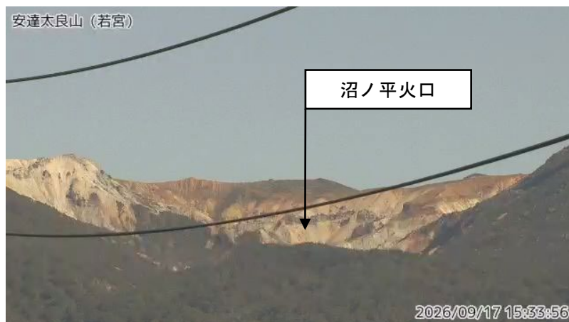
図1 安達太良山 沼ノ平火口周辺の状況（9月17日）
