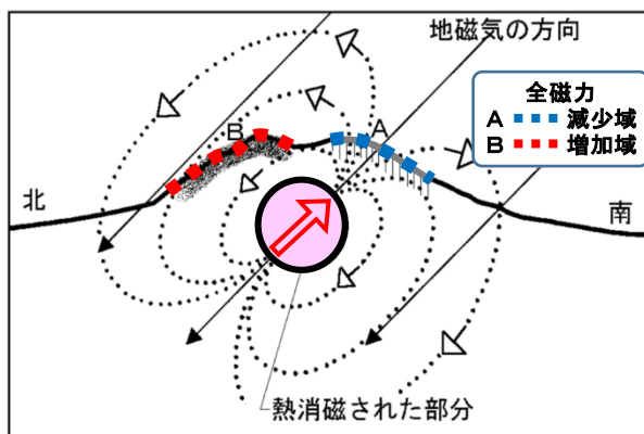
図6 熱消磁に伴う全磁力変化のモデル
