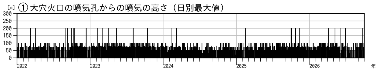
図2 吾妻山 大穴火口の噴気孔からの噴気の高さ（2022年1月～2026年9月）
