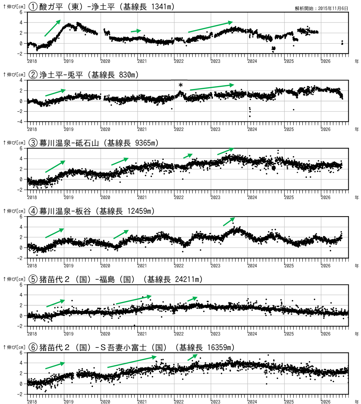
図6 吾妻山 吾妻山浅部・深部の地殻変動（2018年1月～2026年9月）
