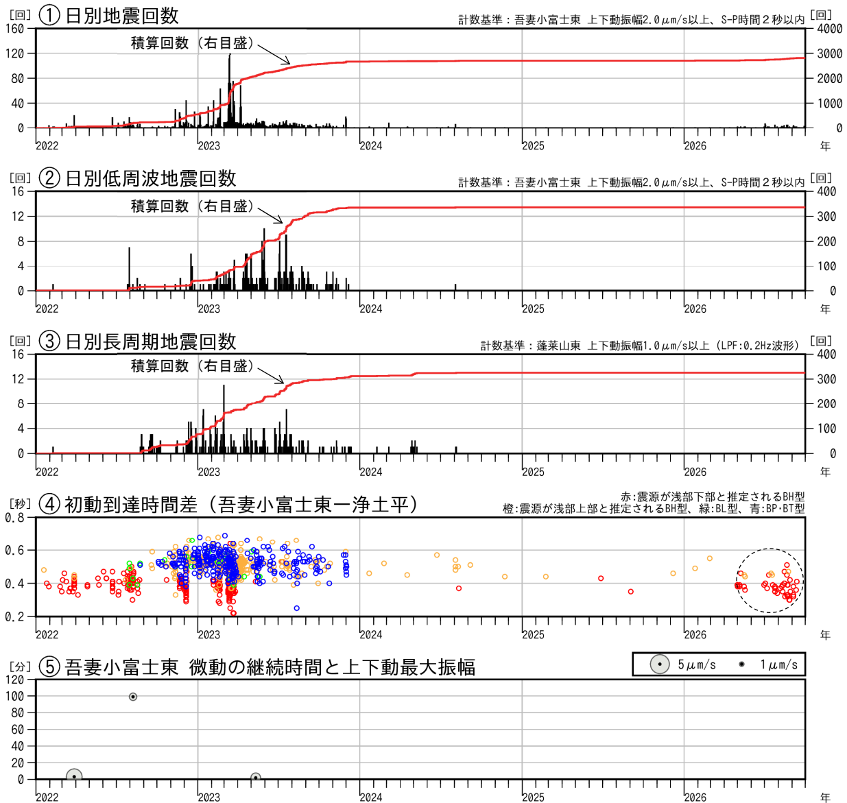
図4 吾妻山 地震活動（2022年1月～2026年9月）
