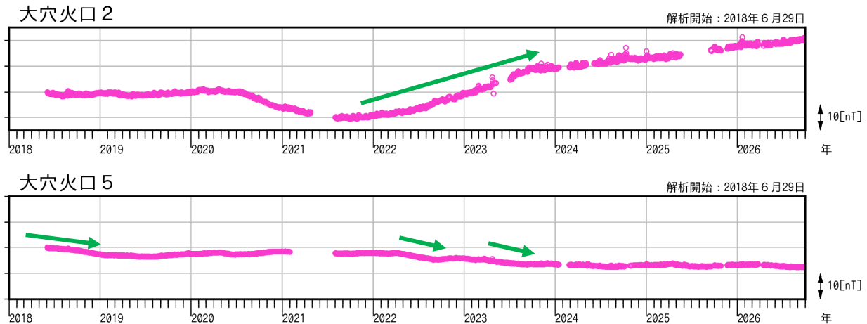
図7 吾妻山 全磁力連続観測点の全磁力値変化（2018年1月～2026年9月）
