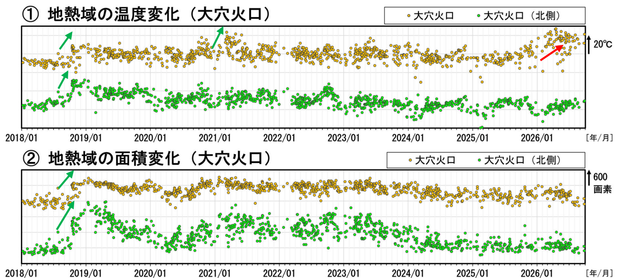
図3-2 吾妻山 監視カメラによる大穴火口周辺の地熱域の経過（2018年1月～2026年9月）
