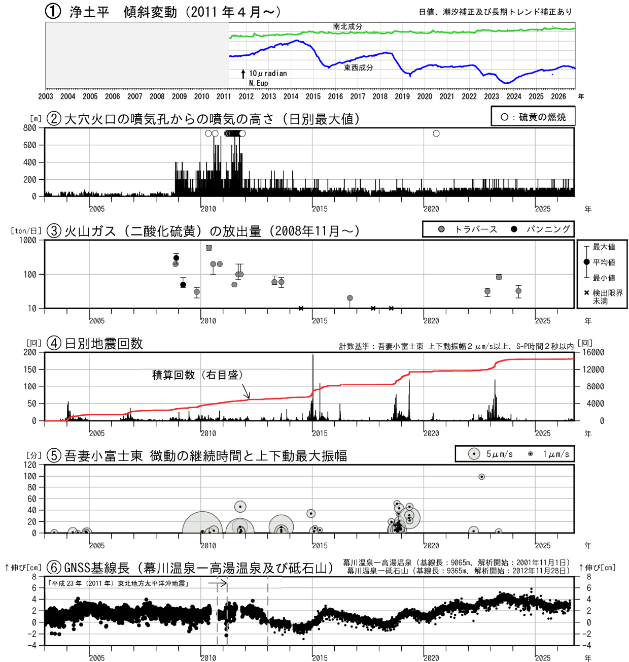
図9 吾妻山 中期的な火山活動の経過（2003年1月～2026年9月）
