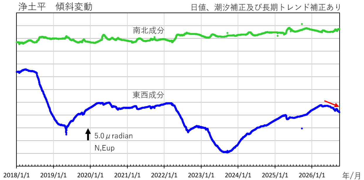
図5 吾妻山 浄土平観測点における傾斜変動（2018年1月～2026年9月）
