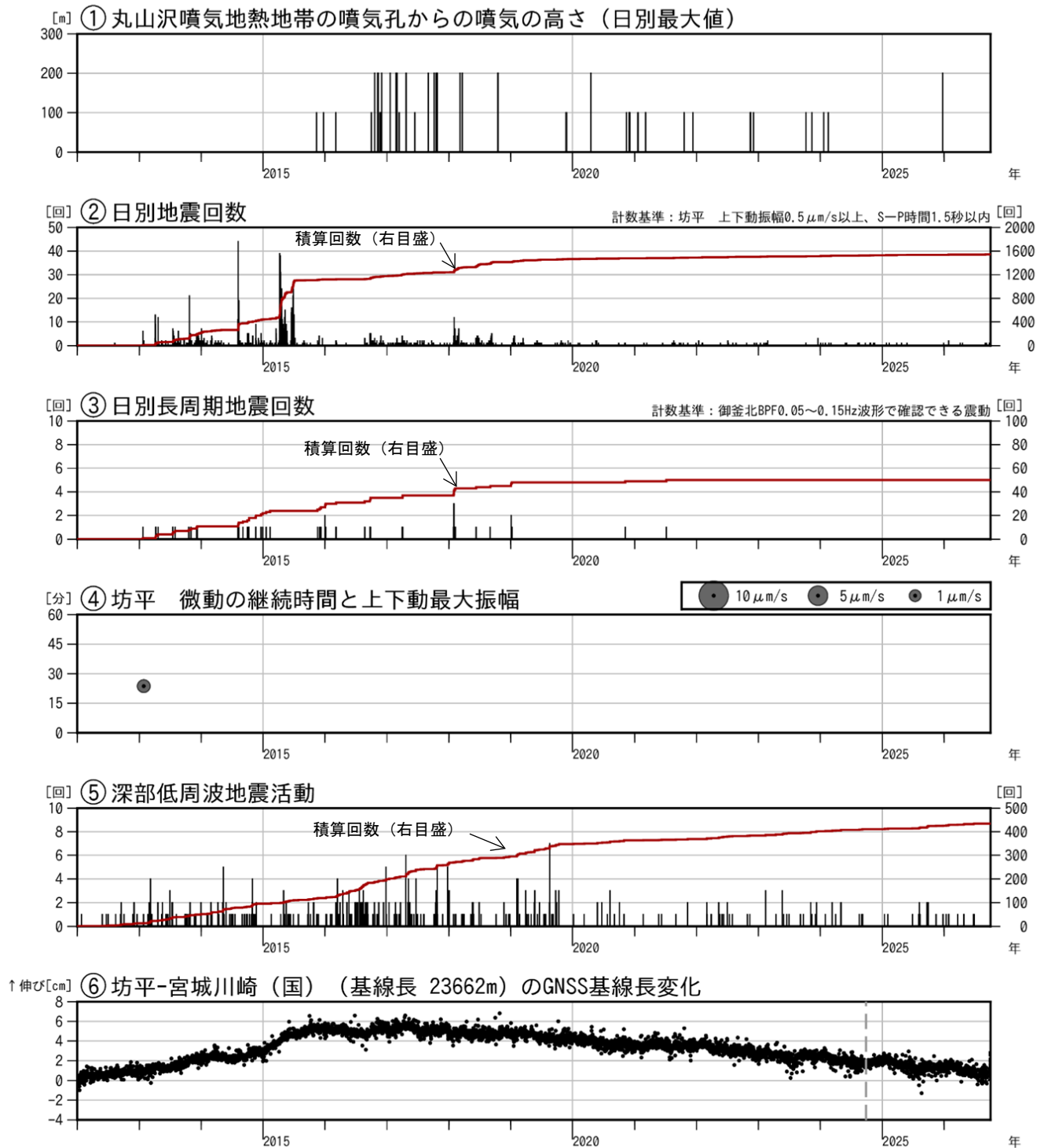
図2 蔵王山 火山活動経過図（2012年1月～2026年9月）
