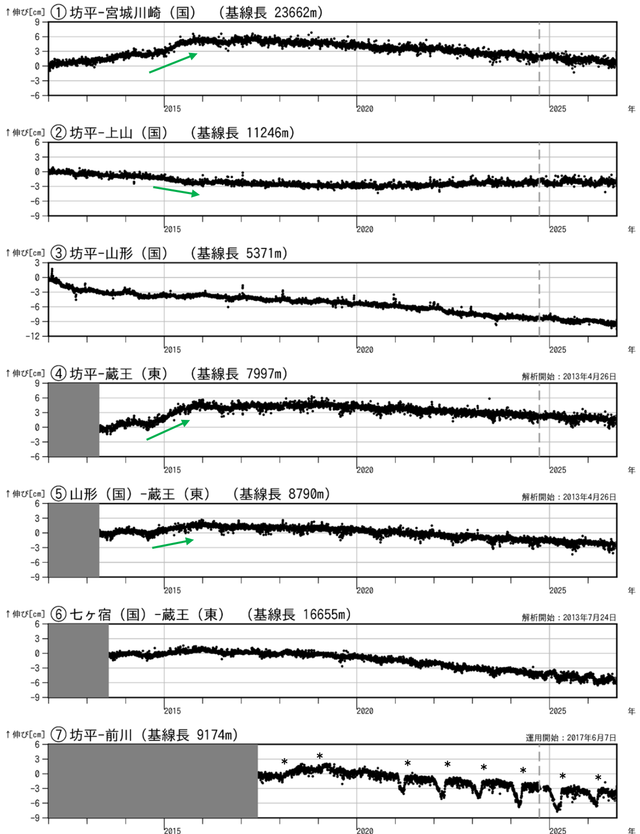
図3 蔵王山 GNSS 基線長変化図 (2012年1月～2026年9月)
