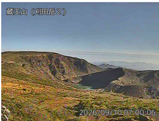
図1 蔵王山 山頂部の状況（9月10日）
