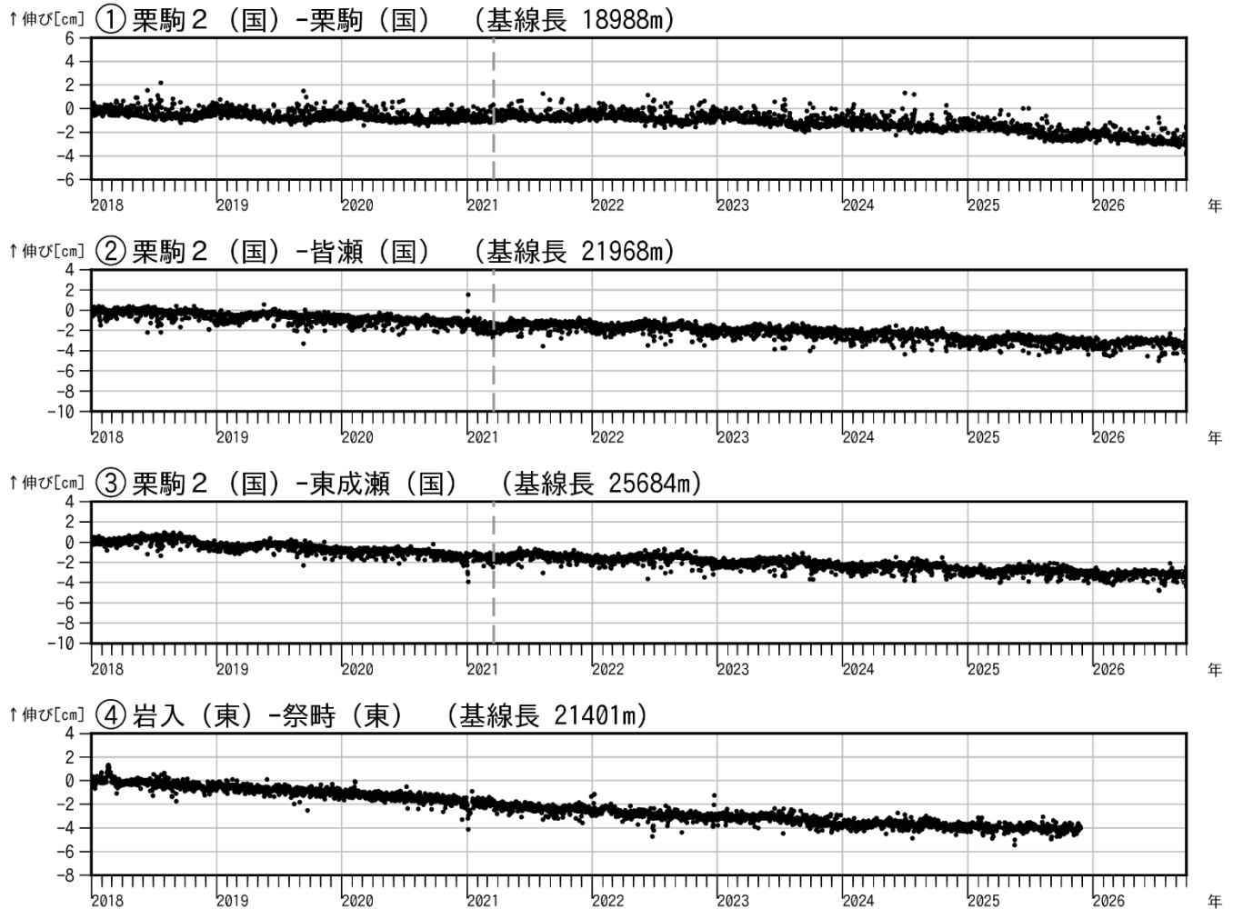
図4 栗駒山 GNSS 基線長変化図（2018年1月～2026年9月）
