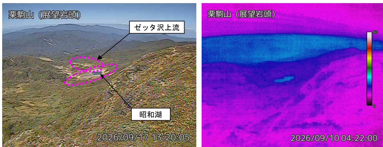
図2 栗駒山 昭和湖及びゼッタ沢上流周辺の状況と地表面温度分布（9月17日（左図）と10日（右図））
