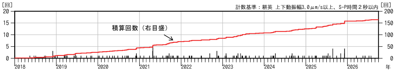
図3 栗駒山 日別地震回数（2018年1月～2026年9月）
