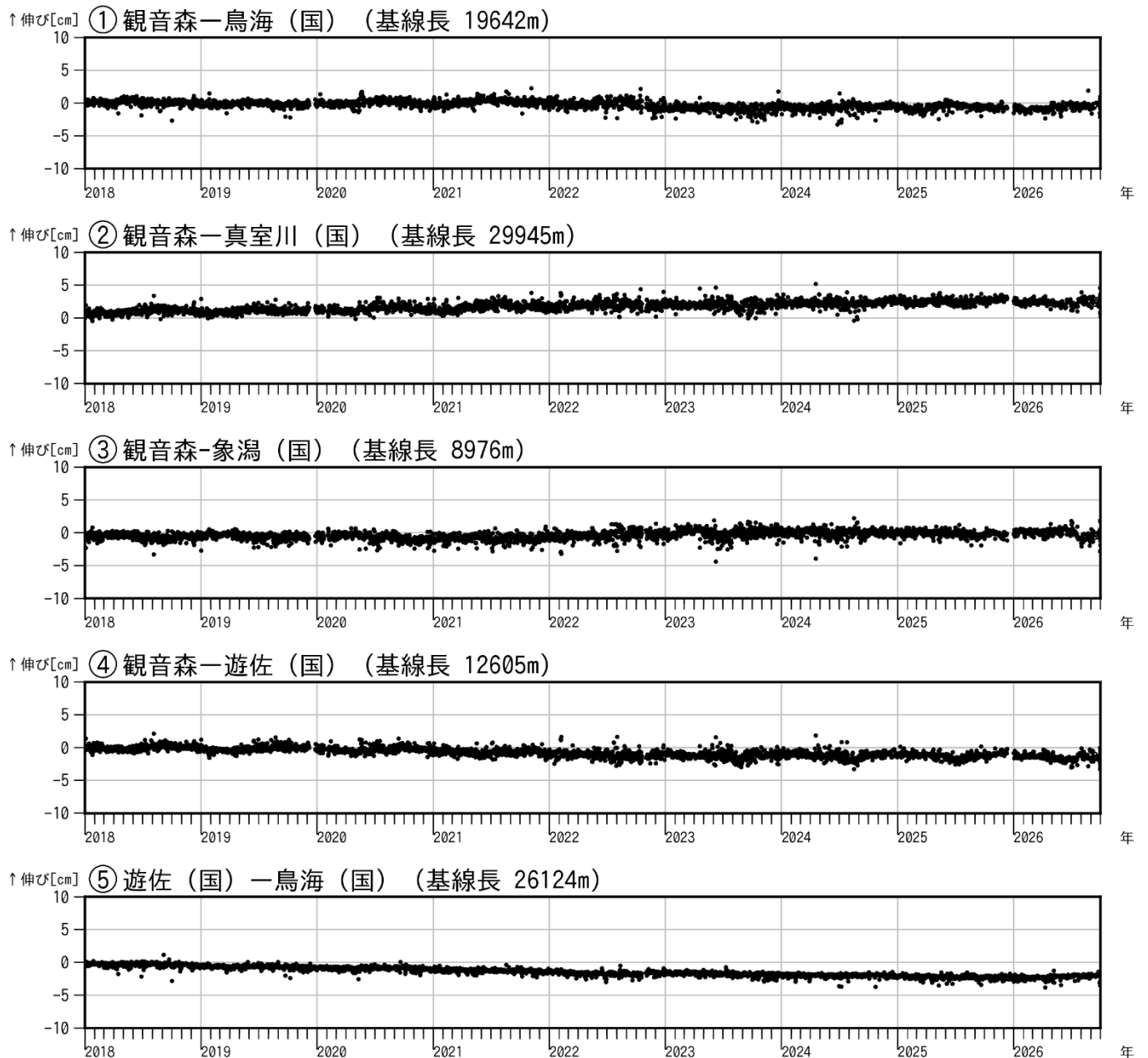
図4 鳥海山 GNSS 基線長変化図（2018年1月～2026年9月）
