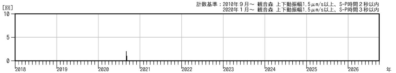
図3 鳥海山 火山性地震の日別回数（2018年1月～2026年9月）
