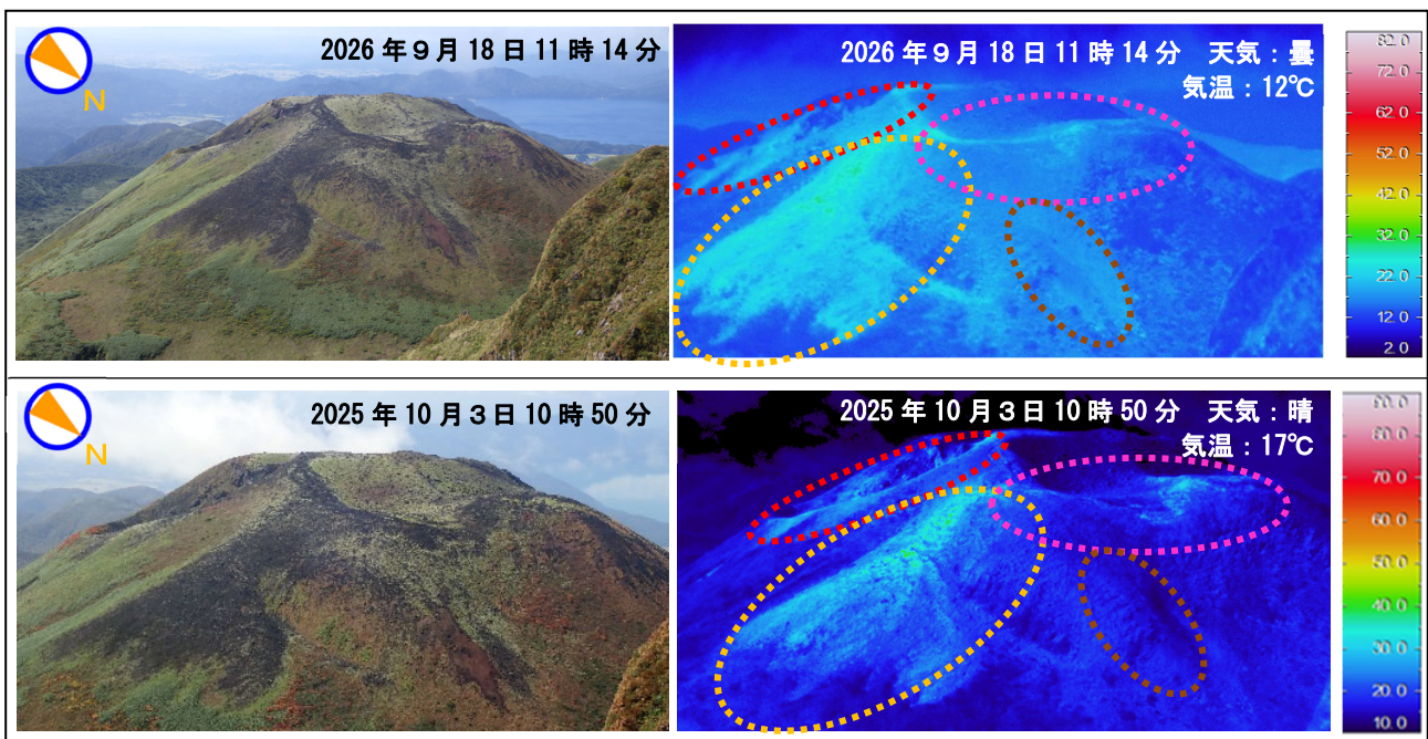
図4 秋田駒ヶ岳 北東方向から撮影した女岳の状況と地表面温度分布
