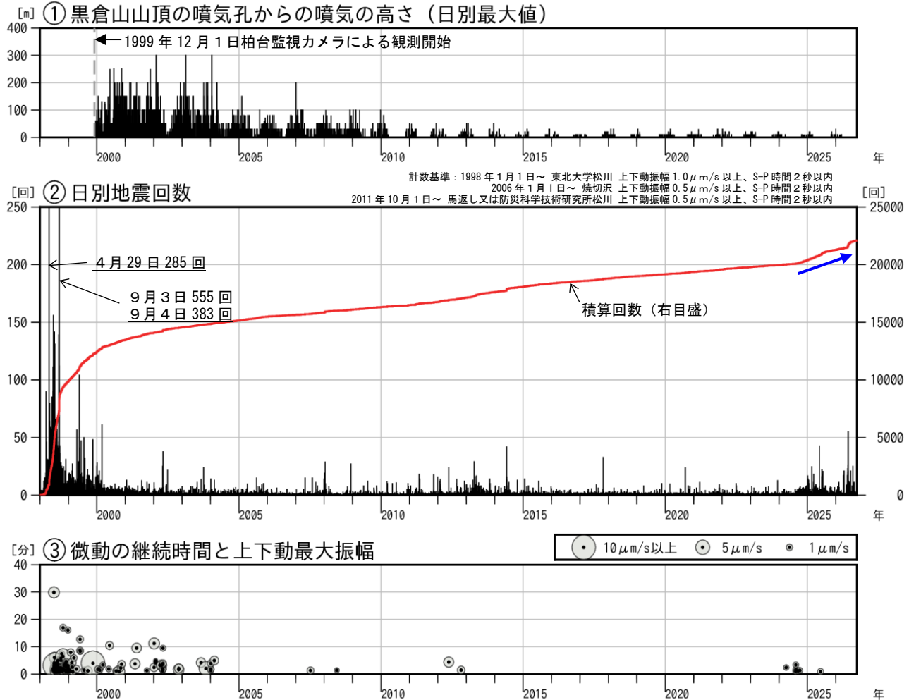
図 1 岩手山 火山活動経過図（1998 年 1 月～2026 年 9 月）
