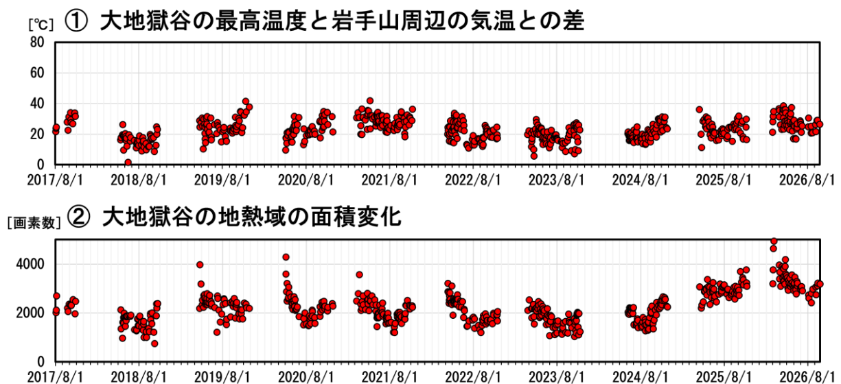
図 5－2 岩手山 黒倉山監視カメラによる大地獄谷の地熱域の経過（2017 年 8 月～2026 年 9 月）
