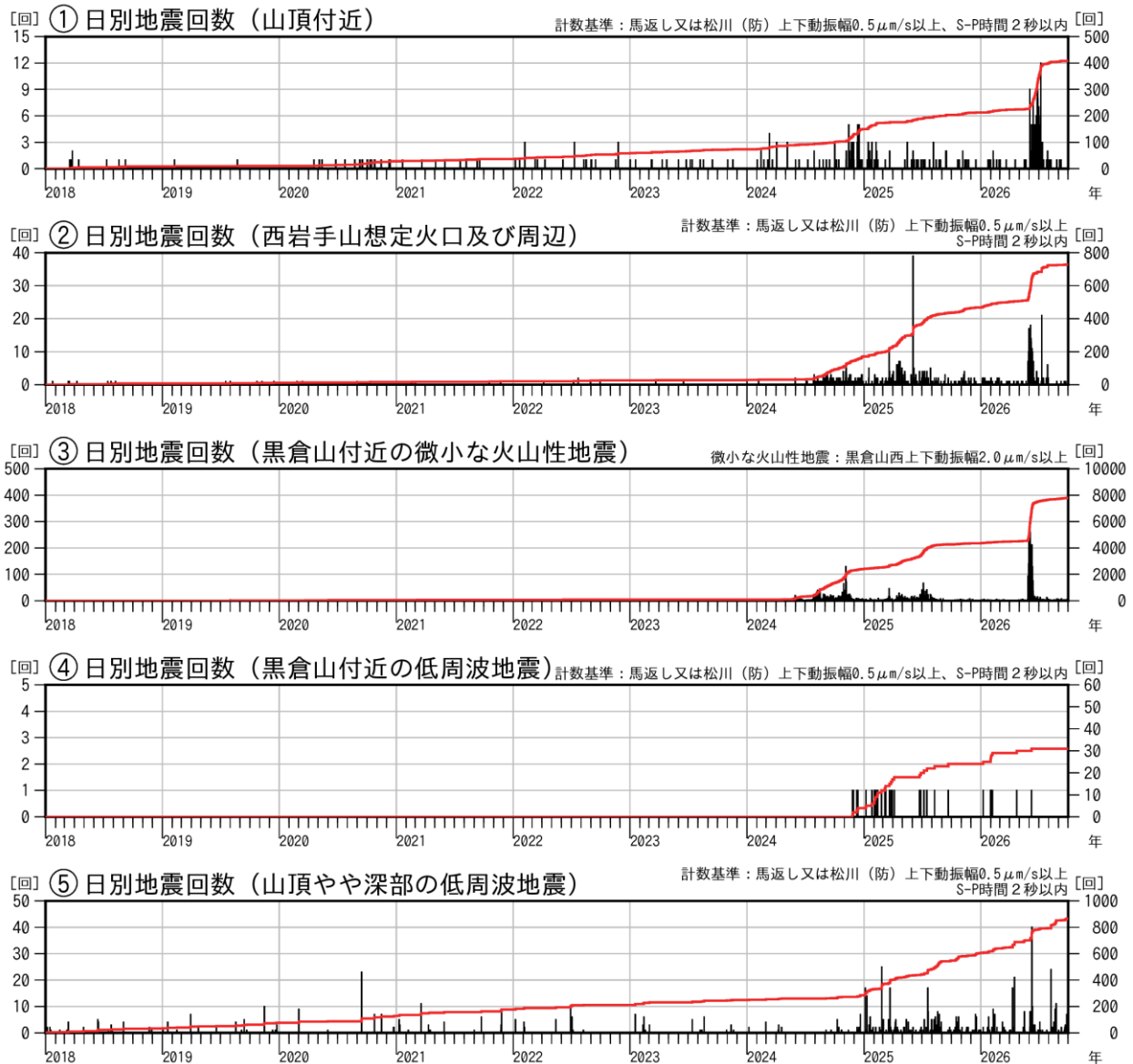
図2 岩手山 日別地震回数（2018年1月～2026年9月）
