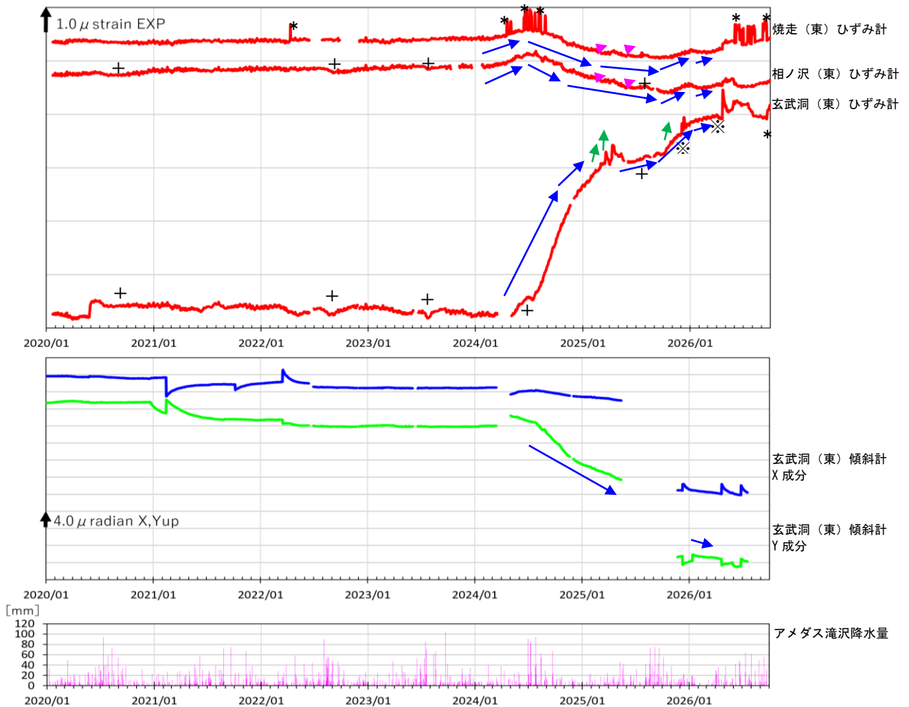
図8 岩手山 ひずみ計・傾斜計（日値・トレンド補正済み）による地殻変動の状況 （2020年1月～2026年9月）
