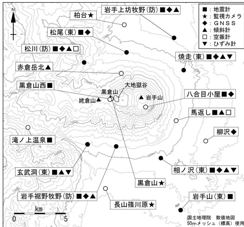
図9 岩手山 観測点配置図
