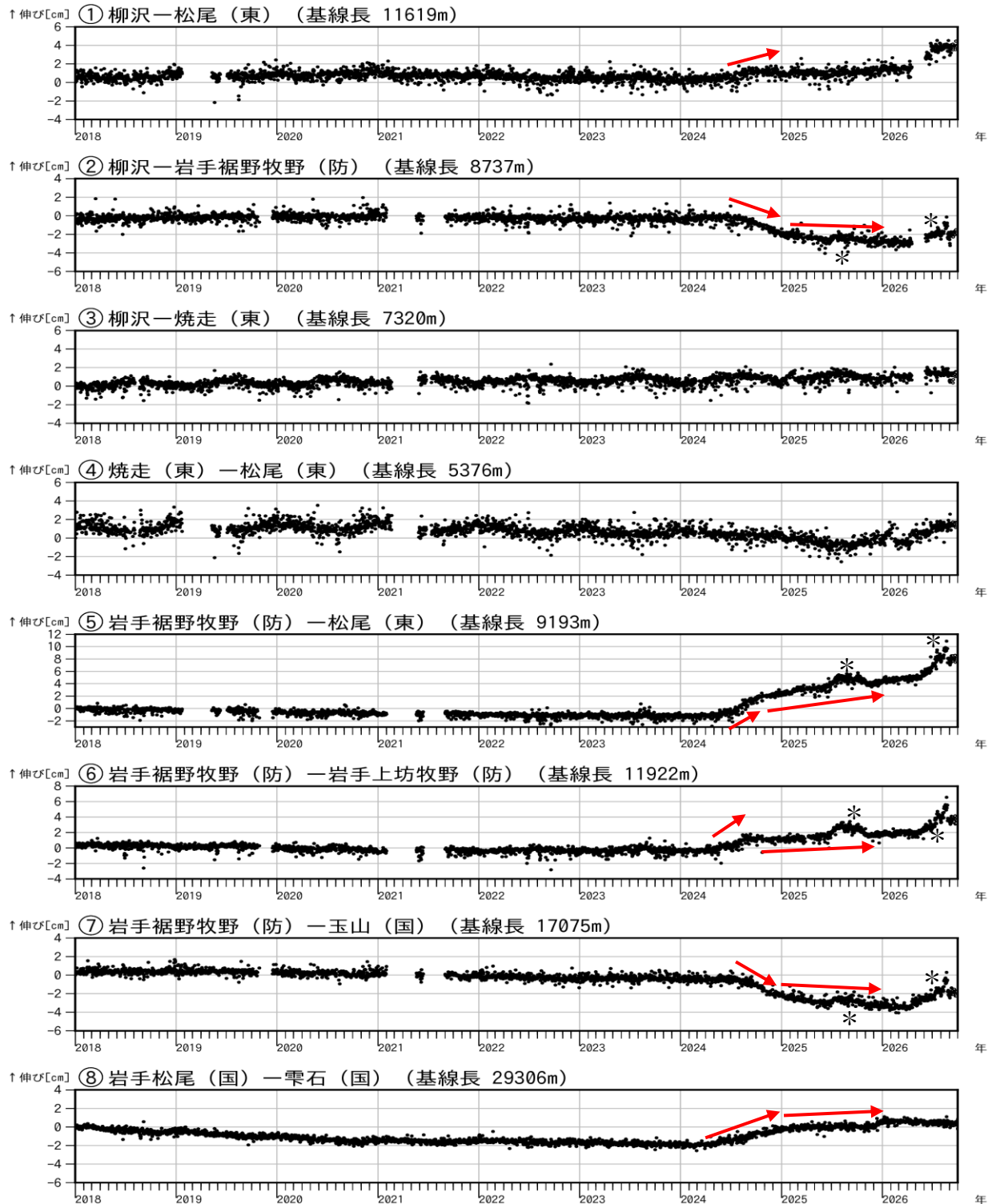
図7 岩手山 GNSS 基線長変化図（2018年1月～2026年9月）
