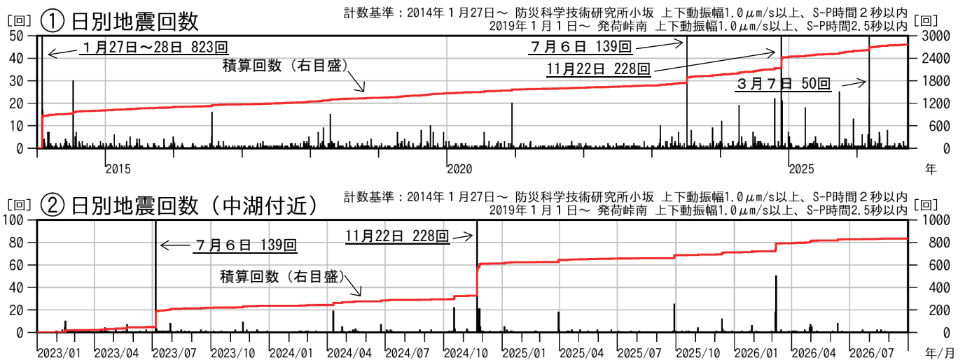
図2 十和田 活動経過図（2014年1月～2026年9月）
