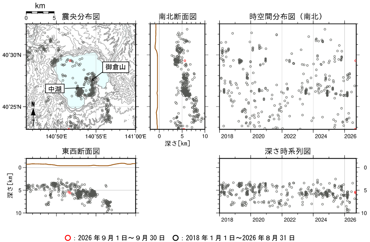
図3 十和田 地震活動（2018年1月～2026年9月）
