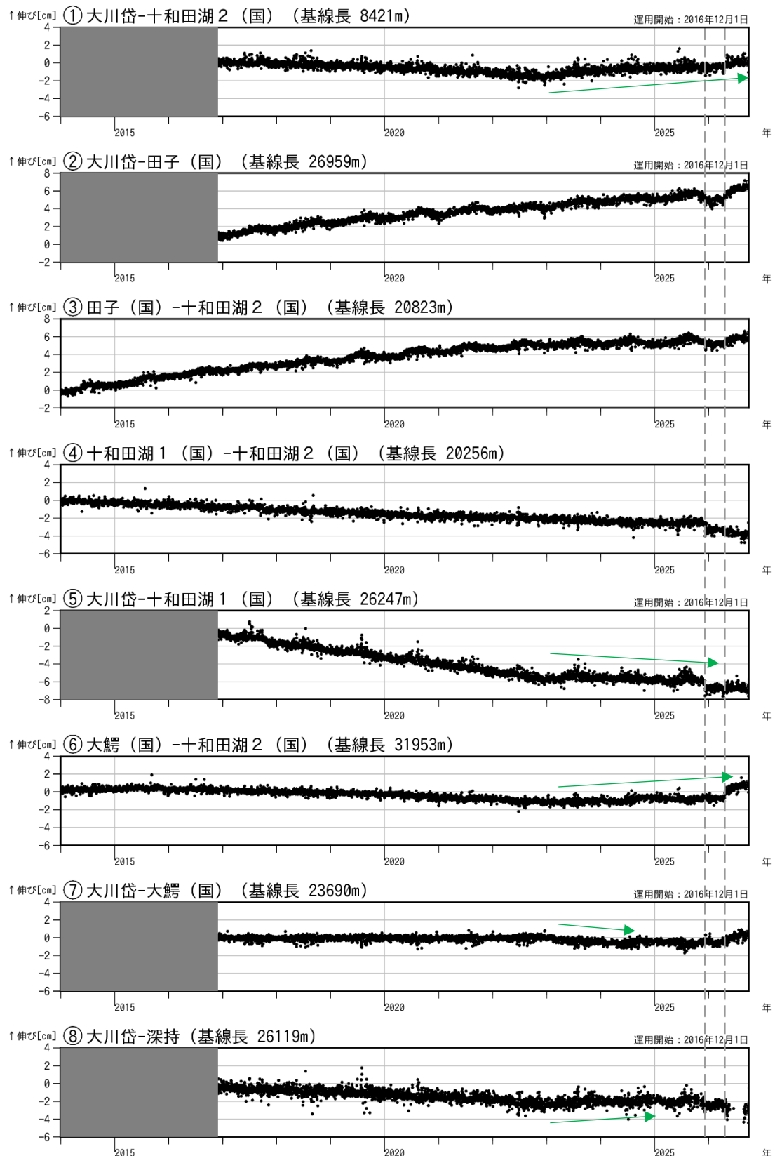
図 4 十和田 GNSS 基線長変化図 (2014 年 1 月～2026 年 9 月)
