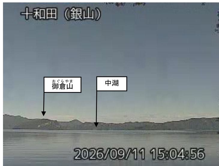
図1 十和田 中湖周辺の状況（9月11日） ・ 銀山監視カメラ（中湖の北西約6 km）の画像です。
