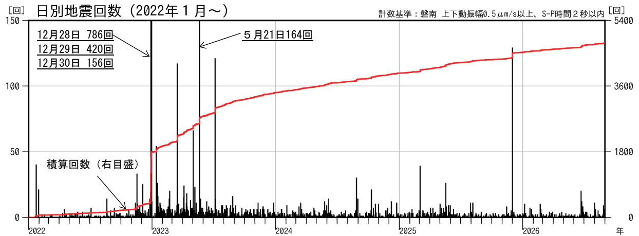
図4 磐梯山 地震回数（2022年1月～2026年8月）
