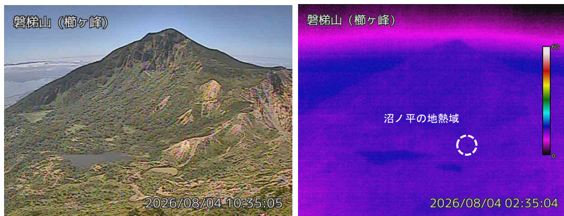
図2 磐梯山 沼ノ平周辺の状況と地表面温度分布（8月4日）
