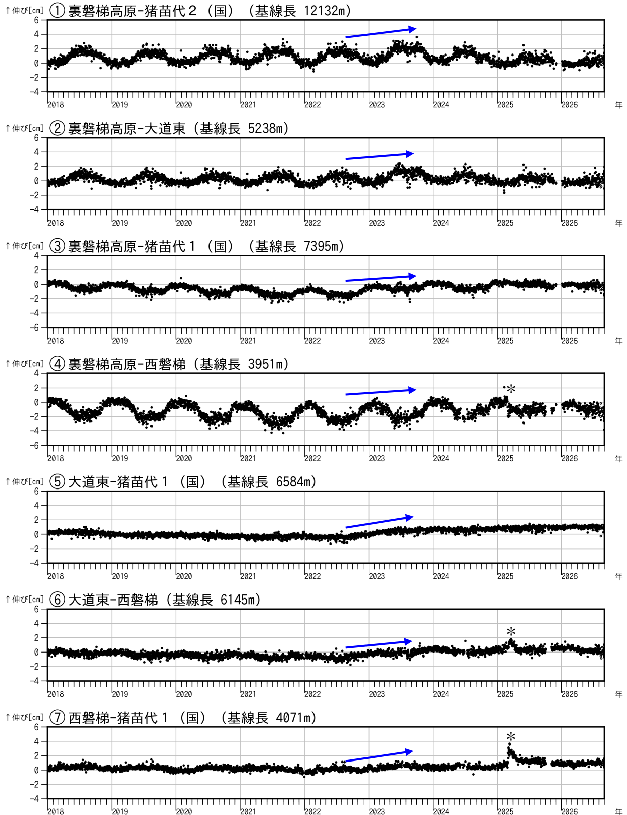
図6 磐梯山 GNSS 基線長変化図（2018年1月～2026年8月）
