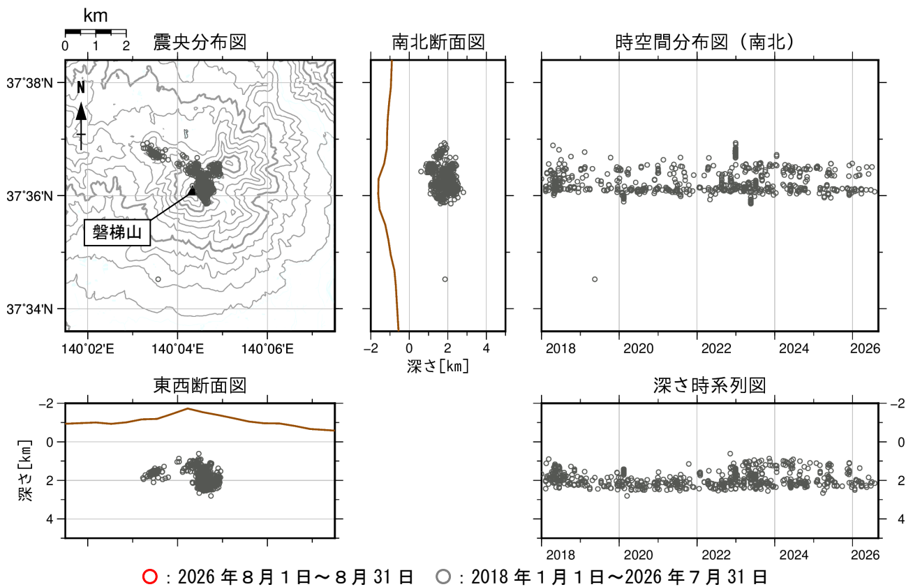
図5 磐梯山 震源分布図（2018年1月～2026年8月）
