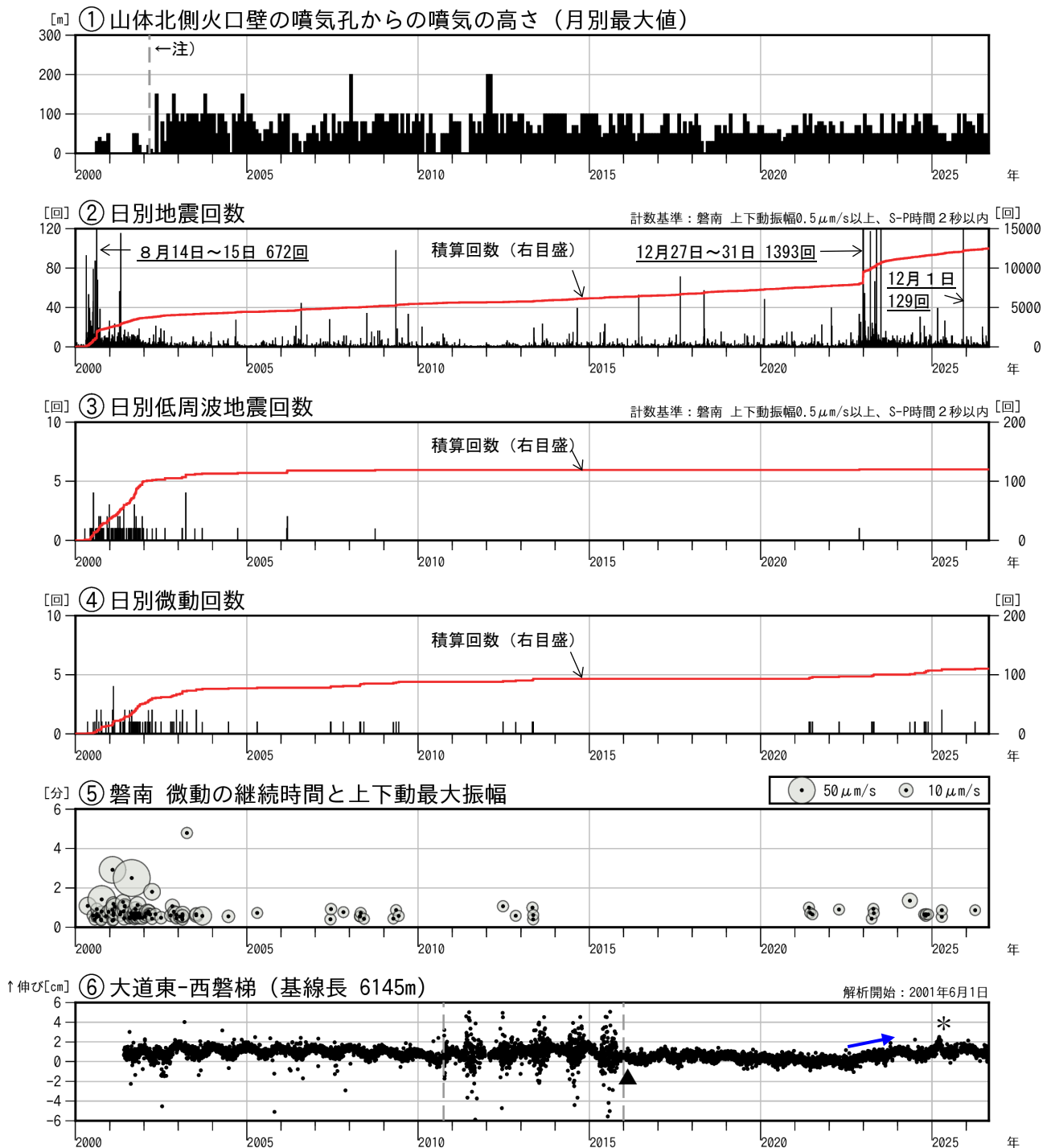
図3 磐梯山 火山活動経過図（2000年1月～2026年8月）
