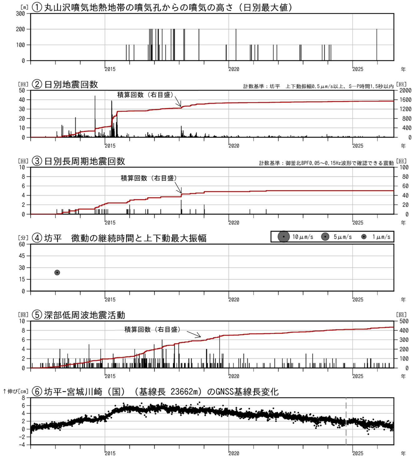
図2 蔵王山 火山活動経過図（2012年1月～2026年8月）
