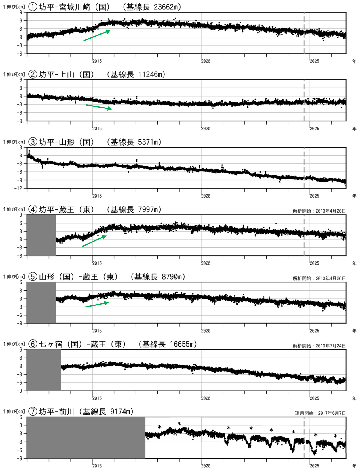
図3 蔵王山 GNSS 基線長変化図 (2012年1月~2026年8月)
