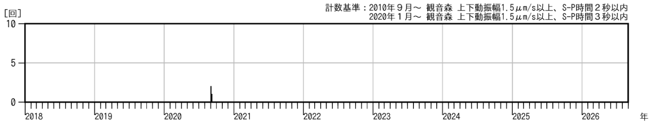
図3 鳥海山 火山性地震の日別回数（2018年1月～2026年8月）
