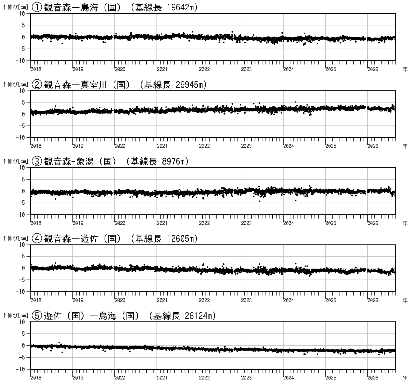
図4 鳥海山 GNSS 基線長変化図（2018年1月～2026年8月）
