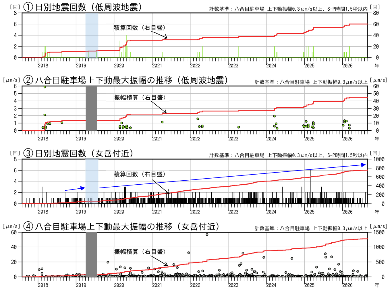
図3 秋田駒ヶ岳 低周波地震及び女岳付近の日別回数と最大振幅（2017年8月～2026年8月）
