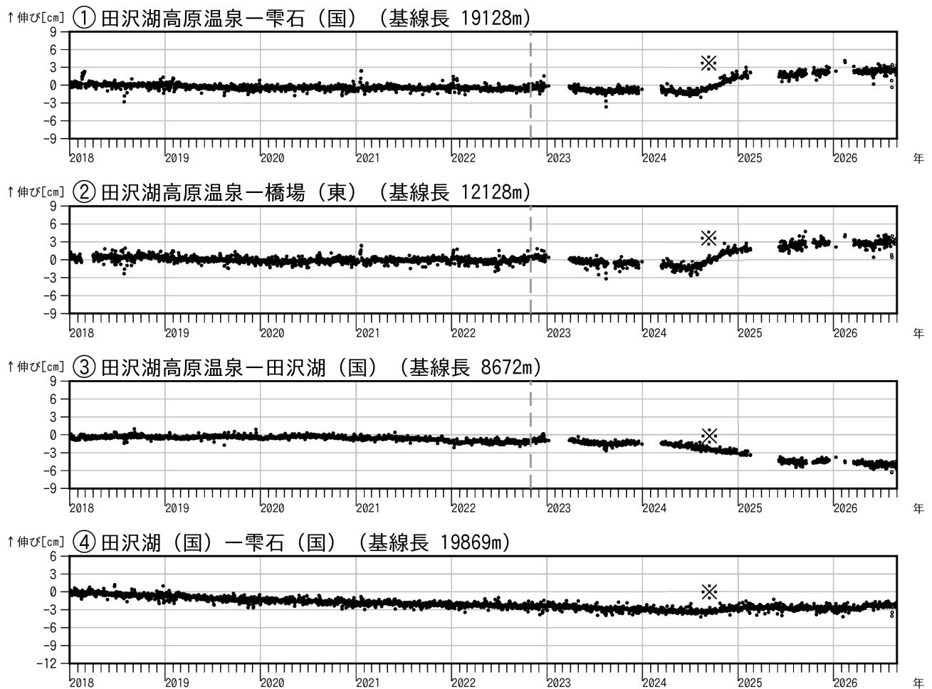
図5 秋田駒ヶ岳 GNSS 基線長変化図（2018年1月～2026年8月）
