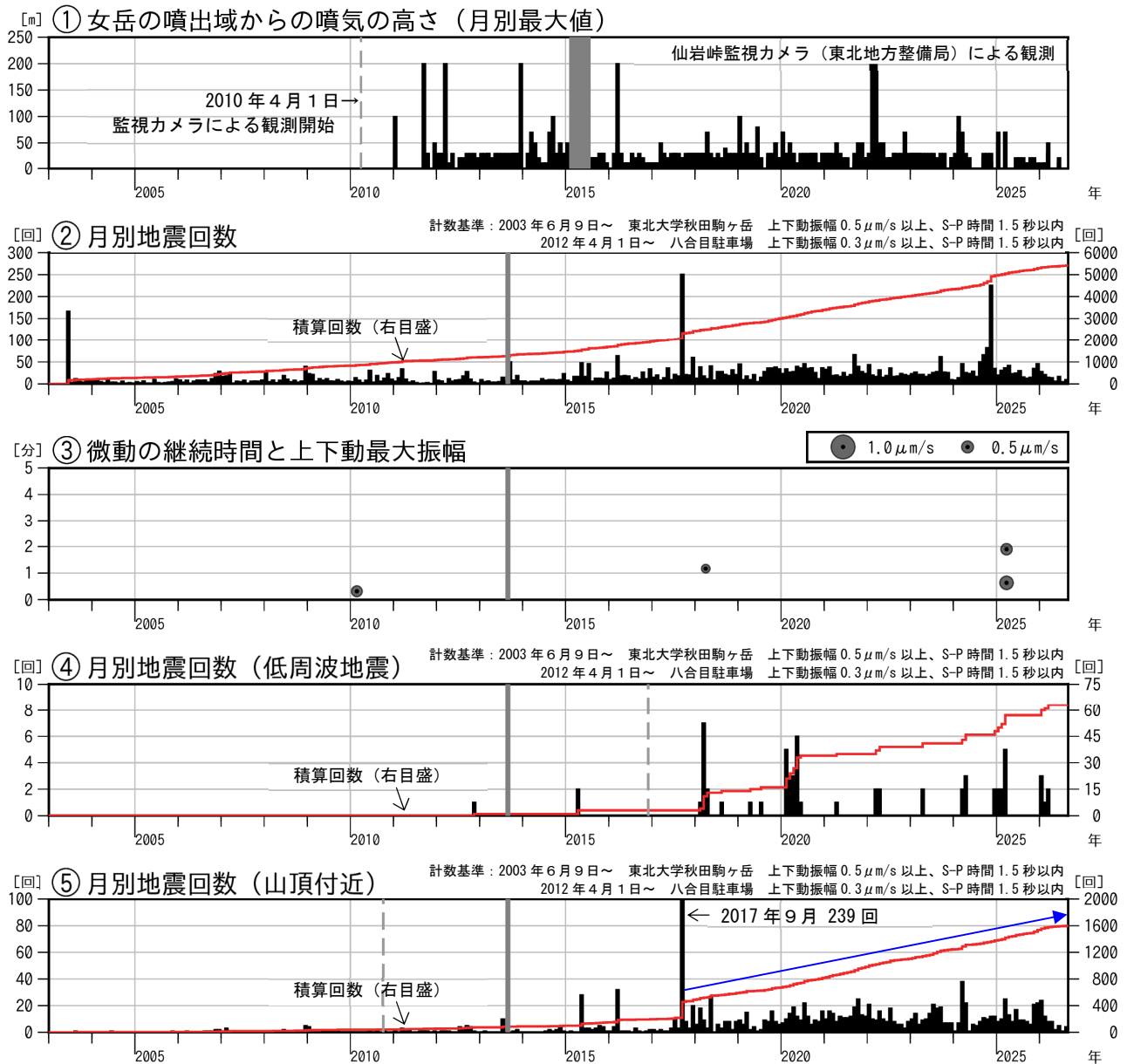
図2 秋田駒ヶ岳 火山活動経過図（2003年6月～2026年8月）
